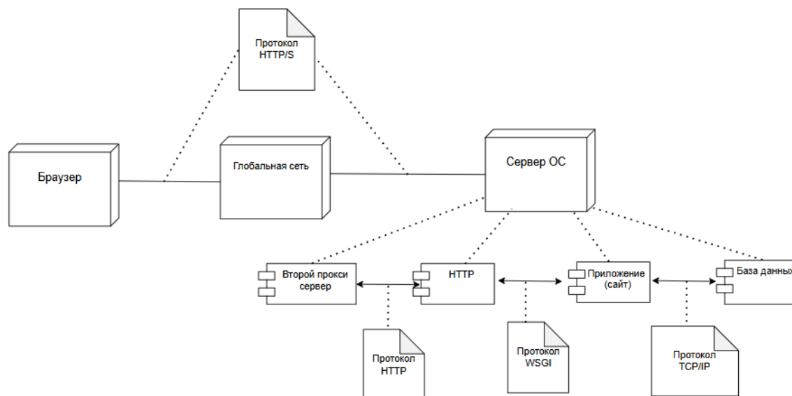
диаграмма развёртывания
