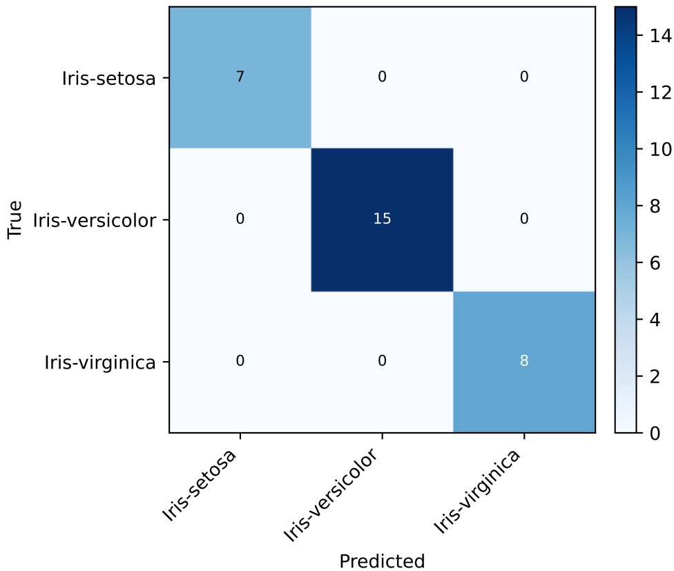
Iris LDA
