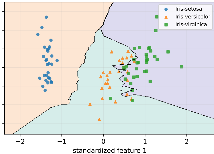
kNN (k=5)
