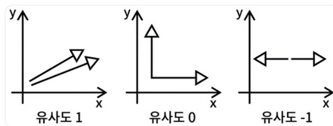
그림 4-6. 코사인 유사도. 각도로 의미 유사도를 측정합니다
