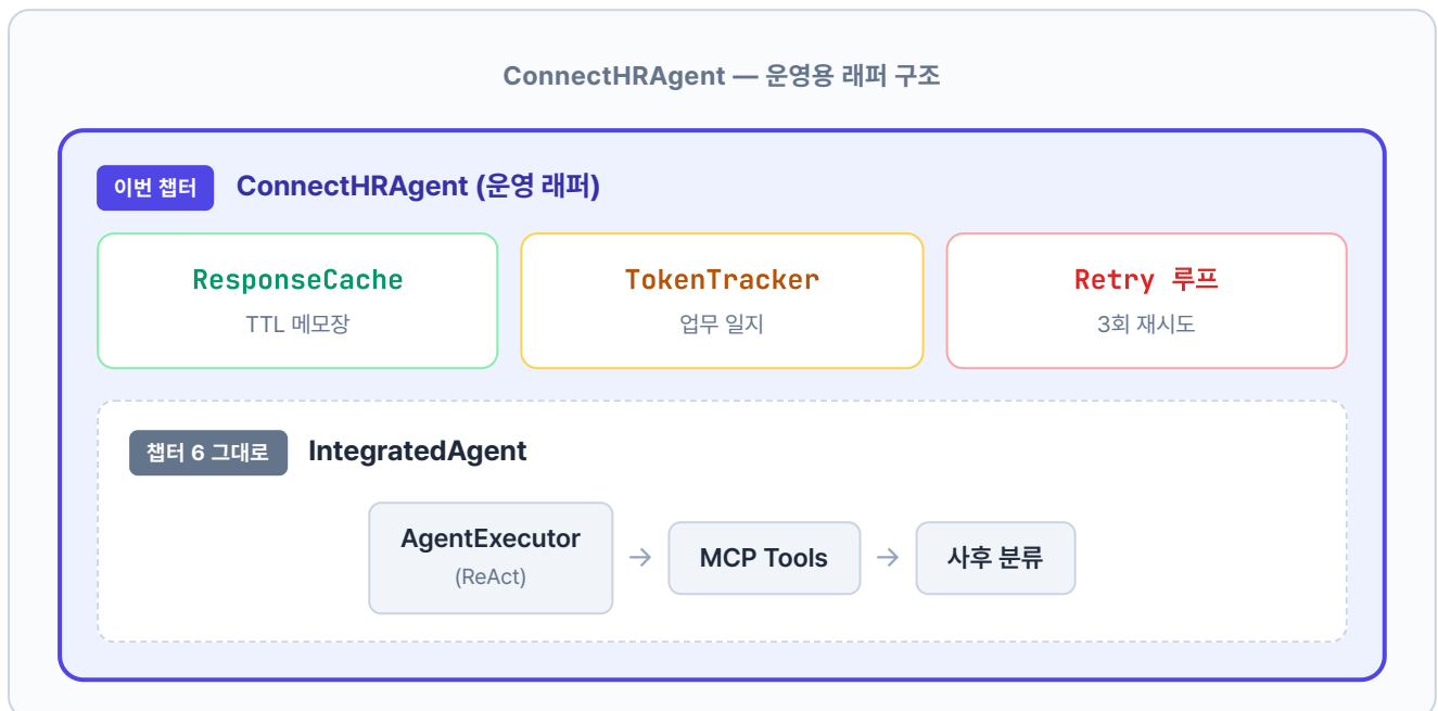
그림 7-6. 챕터 6의 에이전트는 그대로 두고, 바깥을 운영 래퍼 3층 (캐시·추적·재시도)으로 감쌉니다. 요청은 위에서 들어와 래퍼 3층을 거쳐 코어에 닿고, 응답은 반대 방향으로 나오면서 각 층이 추가 작업(저장·기록)을 수행합니다
