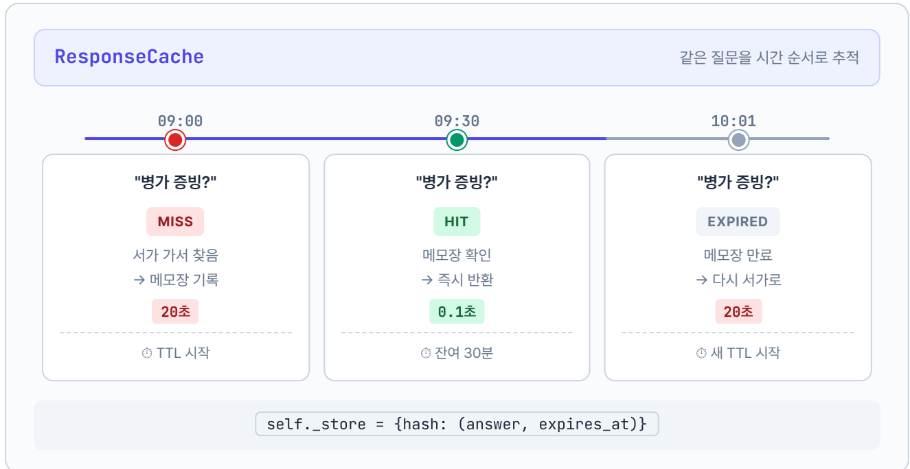
그림 7-4. ResponseCache는 유통기한이 있는 메모장. 같은 질문이 TTL 안에 다시 오면 서가(LLM)를 건너뛴다
