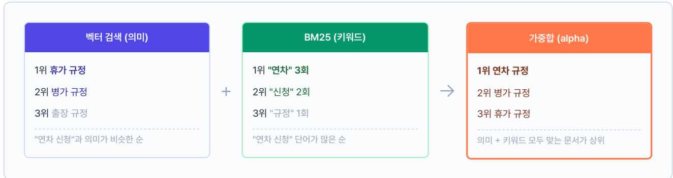
그림 8-11. 하이브리드 검색. 벡터(의미) + BM25(키워드) → 가중치(alpha) 합산
