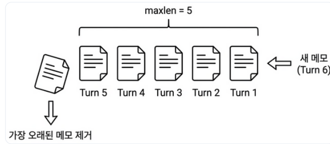
그림 5-4. 6번째 메모가 들어오면 가장 오래된 1번째가 빠집니다. 항상 maxlen = 5
