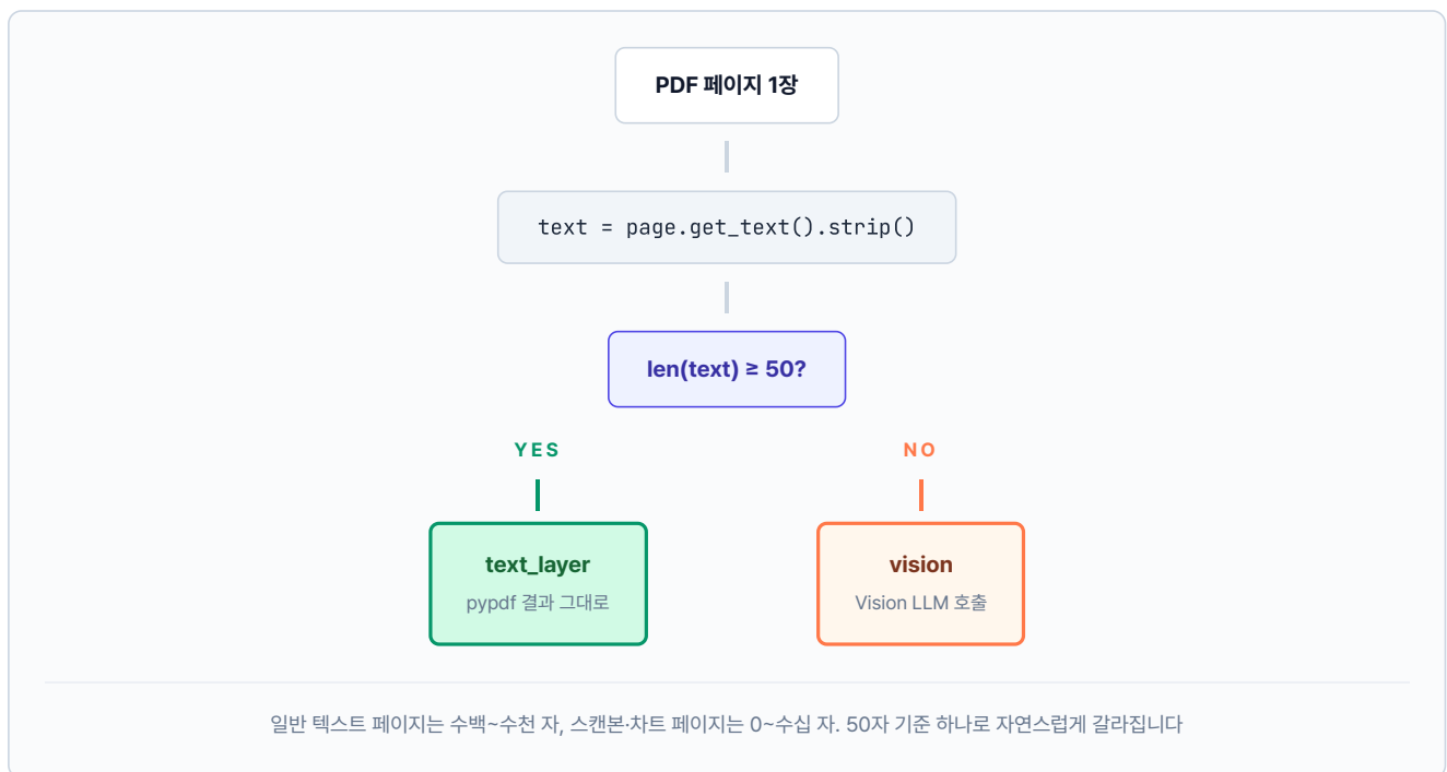
그림 10-7. 하이브리드 파서의 판단 흐름. 페이지마다 텍스트 길이로 분기합니다
