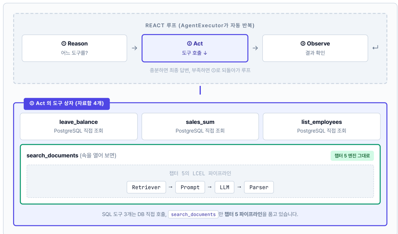
그림 6-4. ReAct 에이전트 안의 파이프라인. 챗터 5 엔진은 버려지지 않고 도구 하나로 감싸져 들어옵니다
