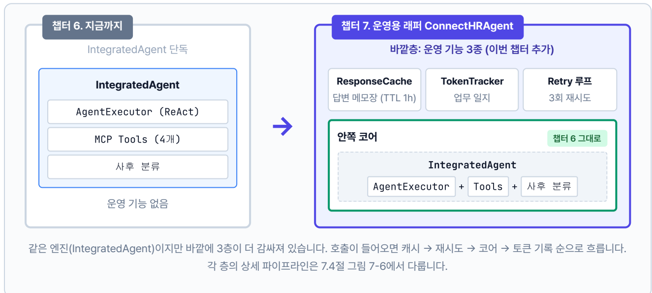
그림 7-2. 챗터 6 에이전트는 그대로, 바깥에 운영 래퍼 3층을 씌웁니다
