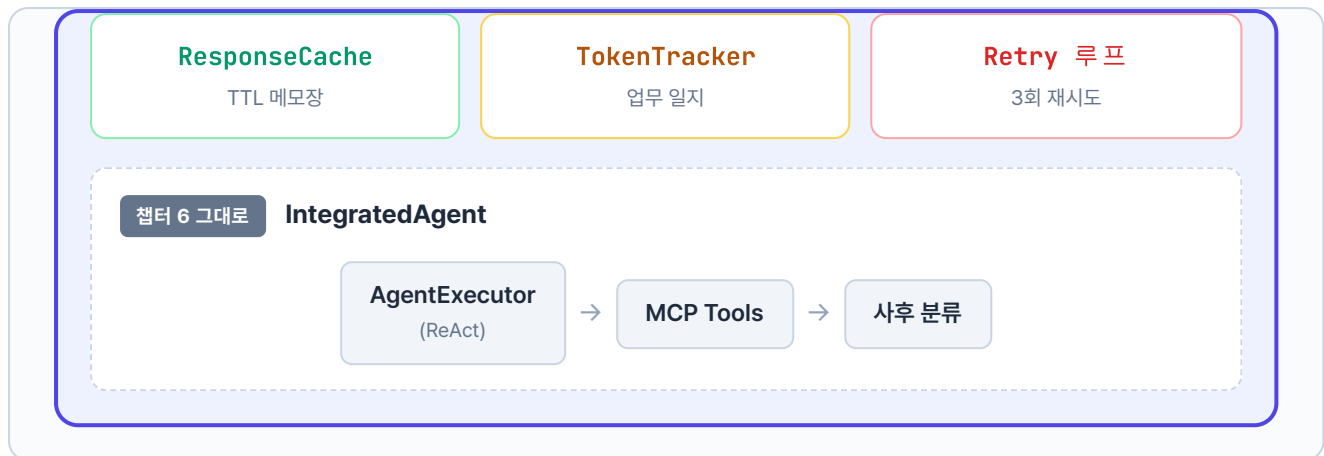
그림 7-6. 챗터 6의 에이전트는 그대로 두고, 바깥을 운영 래퍼 3종 (캐시·추적·재시도)으로 감쌉니다. 요청은 위에서 들어와 래퍼 3층을 거쳐 코어에 닿고, 응답은 반대 방향으로 나오면서 각 층이 추가 작업(저장·기록)을 수행합니다
