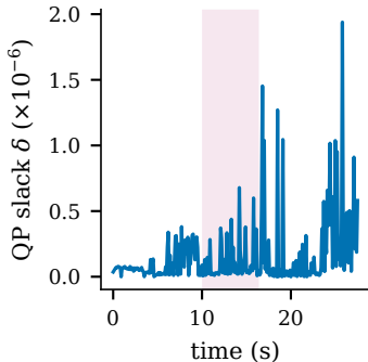
(d) QP slack stays \approx 0
