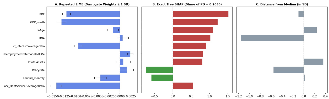
Figure 22: ผลการอธิบายความเสี่ยงด้วย LIME และ SHAP ของบริษัท PRIME (งวด 2025-11)
