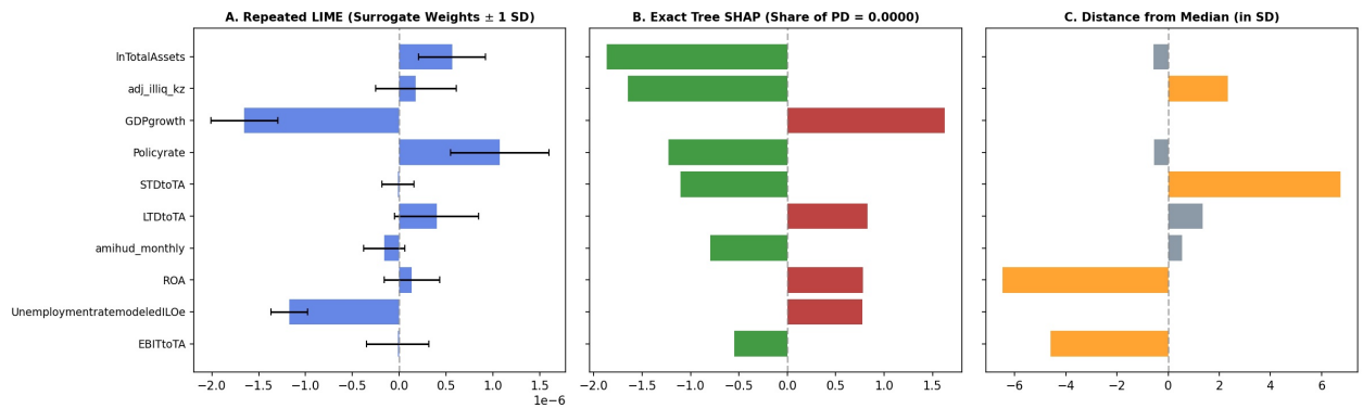
Figure 15: ผลการอธิบายความเสี่ยงด้วย LIME และ SHAP ของบริษัท CHO (งวด 2026-08)
