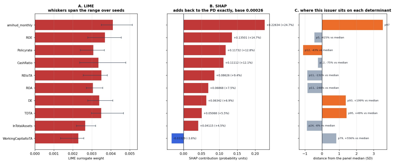
Figure 5: ผลการอธิบายความเสี่ยงด้วย LIME และ SHAP ของบริษัท CI (งวด 2026-08)
