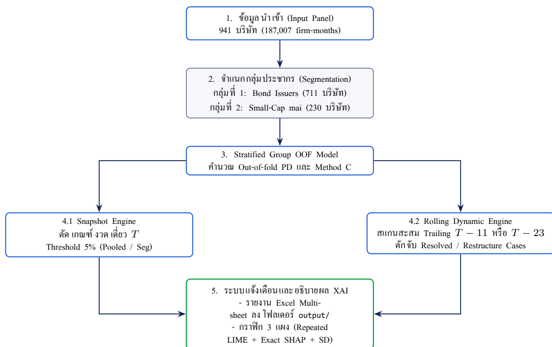
Figure 2: แผนผังโครงสร้างสถาปัตยกรรมการตรวจจับความเสี่ยงและอธิบายผลทั้ง 6 รูปแบบ
