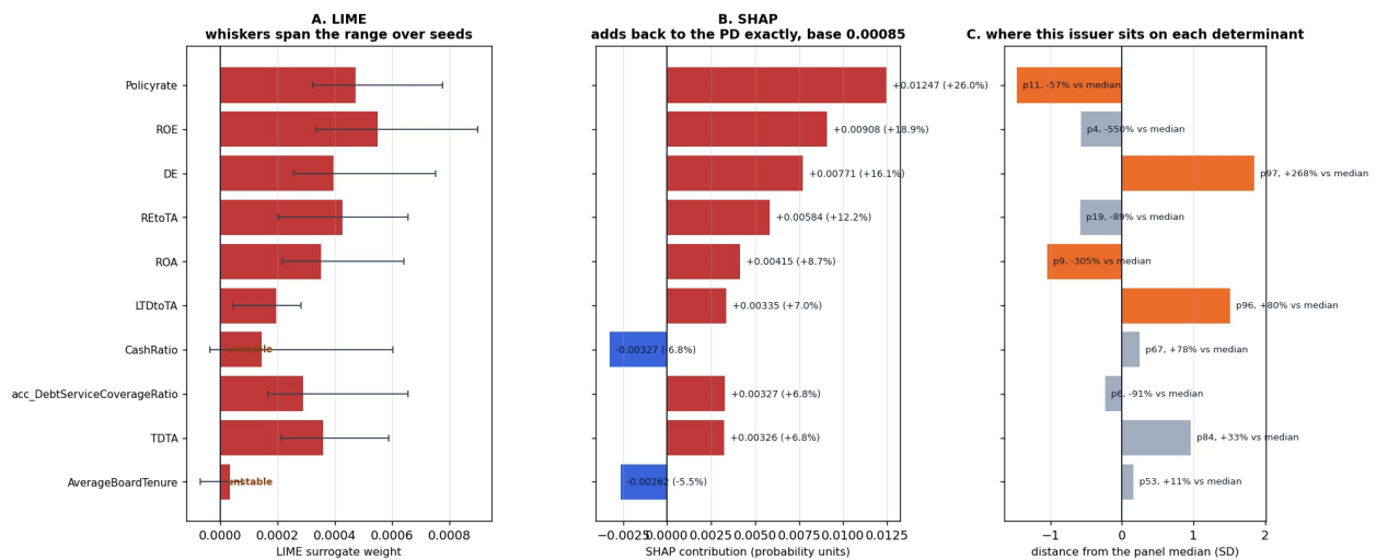
Figure 19: ผลการอธิบายความเสี่ยงด้วย LIME และ SHAP ของบริษัท DTP (งวด 2026-08)
