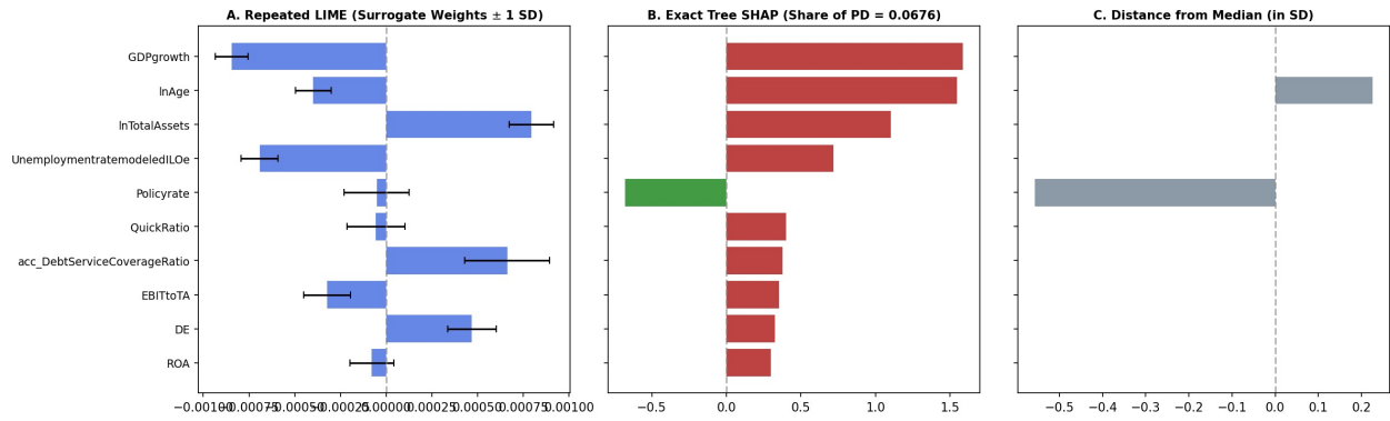
Figure 21: ผลการอธิบายความเสี่ยงด้วย LIME และ SHAP ของบริษัท ECF (งวด 2026-03)
