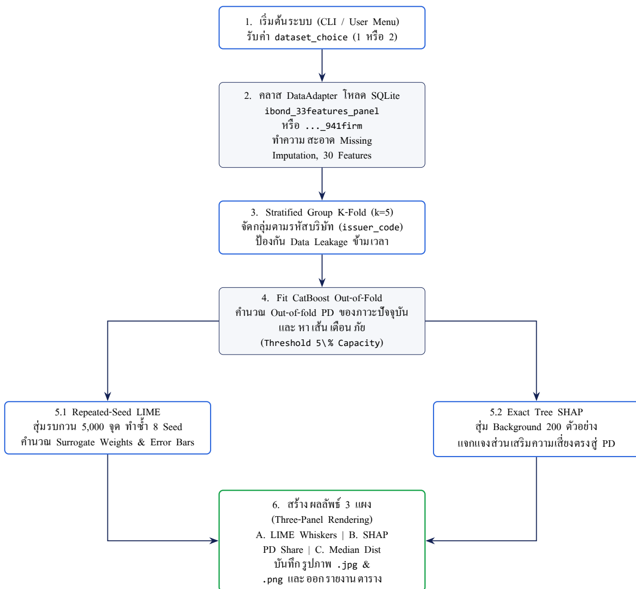
Figure 1: แผนผังขั้นตอนอัลกอริทึมของระบบ DataAdapter และ XAI Engine (LIME & SHAP)
