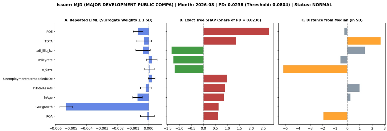
Figure 3: ผลการอธิบายความเสี่ยงด้วย LIME และ SHAP ของบริษัท MJD (งวด 2026-08)
