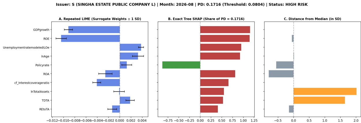
Figure 12: ผลการอธิบายความเสี่ยงด้วย LIME และ SHAP ของบริษัท S (งวด 2026-08)
