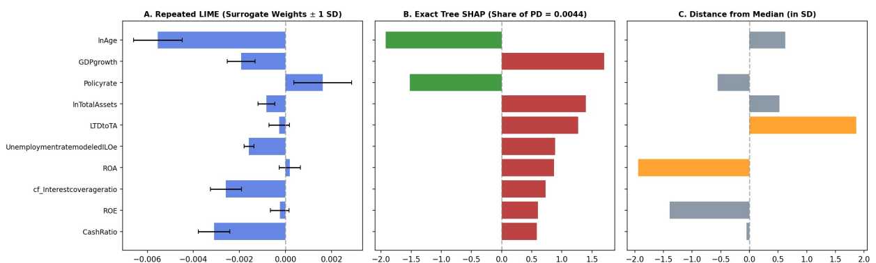
Figure 6: ผลการอธิบายความเสี่ยงด้วย LIME และ SHAP ของบริษัท TPOLY (งวด 2026-06)
