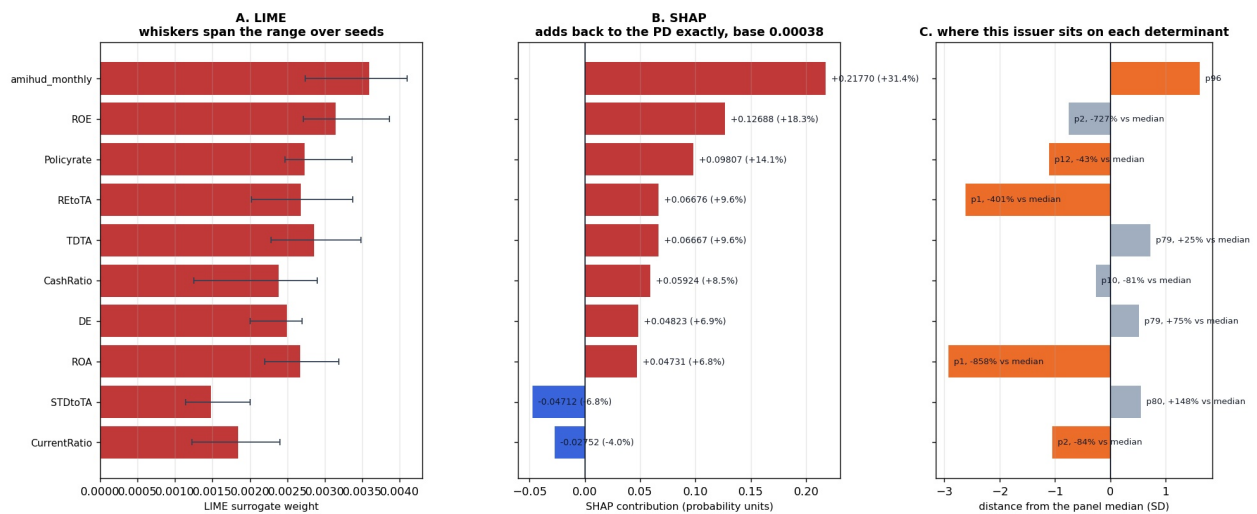
Figure 7: ผลการอธิบายความเสี่ยงด้วย LIME และ SHAP ของบริษัท MUD (งวด 2026-08)
