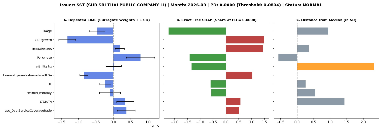
Figure 13: ผลการอธิบายความเสี่ยงด้วย LIME และ SHAP ของบริษัท SST (งวด 2026-08)
