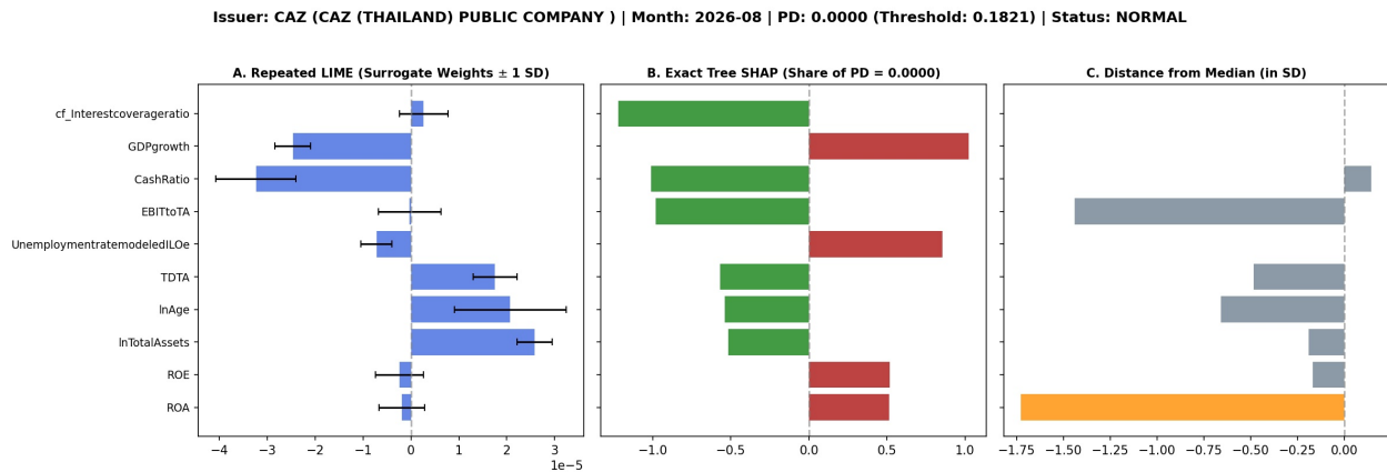
Figure 17: ผลการอธิบายความเสี่ยงด้วย LIME และ SHAP ของบริษัท CAZ (งวด 2026-08)
