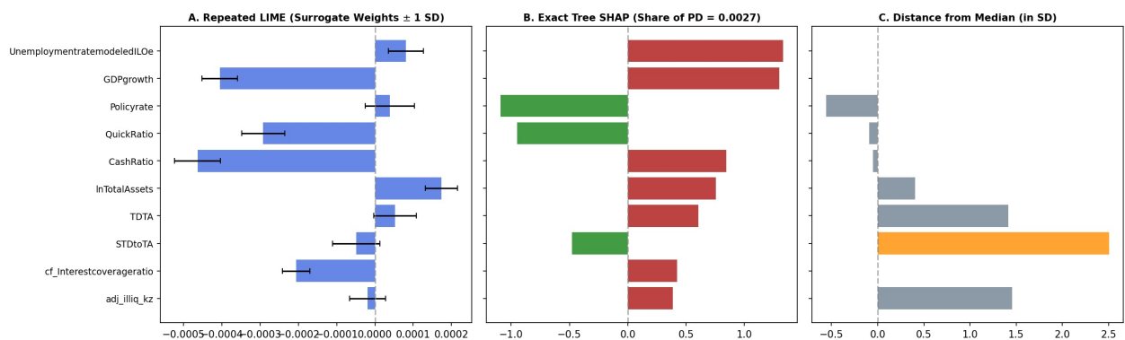
Figure 20: ผลการอธิบายความเสี่ยงด้วย LIME และ SHAP ของบริษัท RML (งวด 2026-08)
