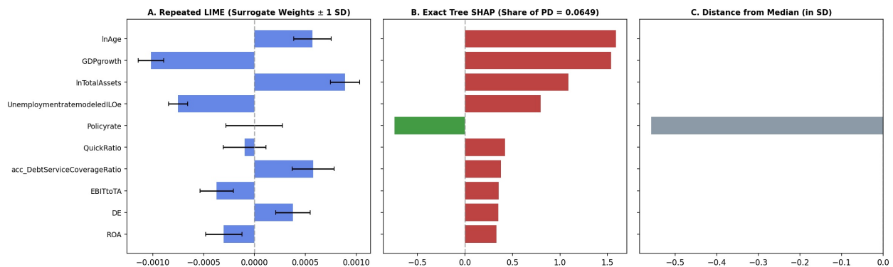
Figure 16: ผลการอธิบายความเสี่ยงด้วย LIME และ SHAP ของบริษัท GRAND (งวด 2026-03)
