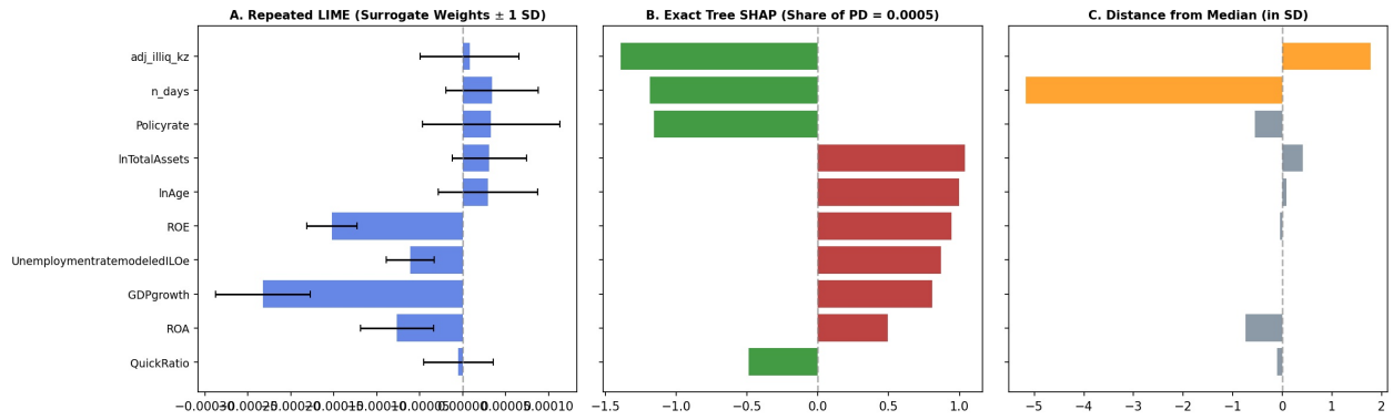
Figure 14: ผลการอธิบายความเสี่ยงด้วย LIME และ SHAP ของบริษัท RICHY (งวด 2026-08)
