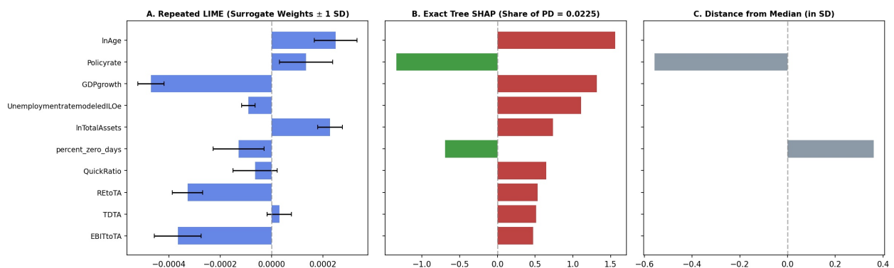
Figure 8: ผลการอธิบายความเสี่ยงด้วย LIME และ SHAP ของบริษัท NRF (งวด 2026-08)
