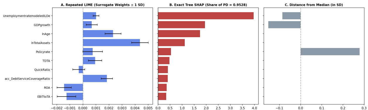
Figure 11: ผลการอธิบายความเสี่ยงด้วย LIME และ SHAP ของบริษัท NWR (งวด 2026-08)
