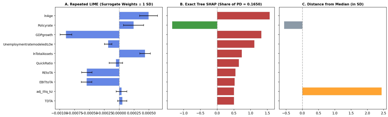
Figure 9: ผลการอธิบายความเสี่ยงด้วย LIME และ SHAP ของบริษัท PF (งวด 2026-05)
