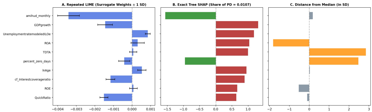
Figure 10: ผลการอธิบายความเสี่ยงด้วย LIME และ SHAP ของบริษัท A (งวด 2026-01)
