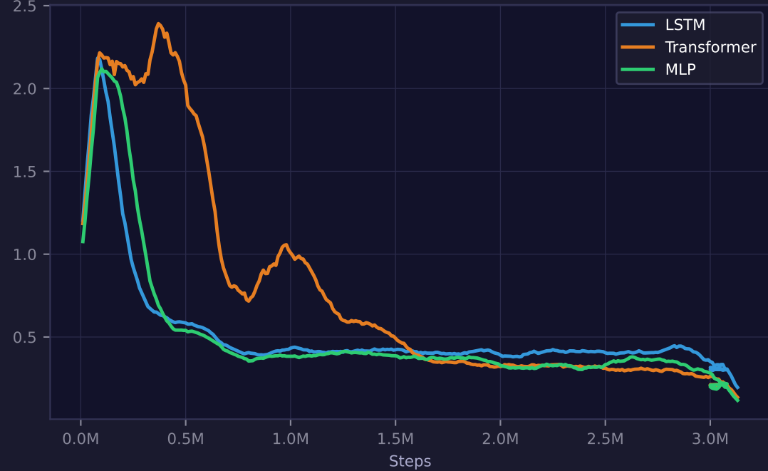
Distanz-Fortschritt [%] (Start→Ende)
