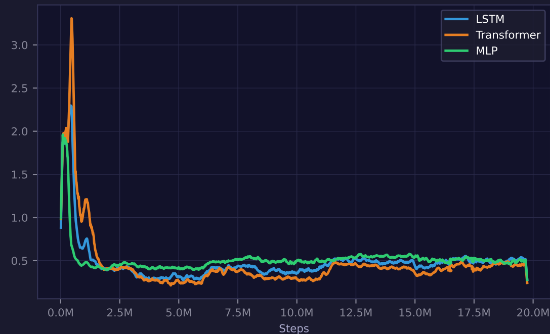
Distanz-Fortschritt [%] (Start→Ende)
