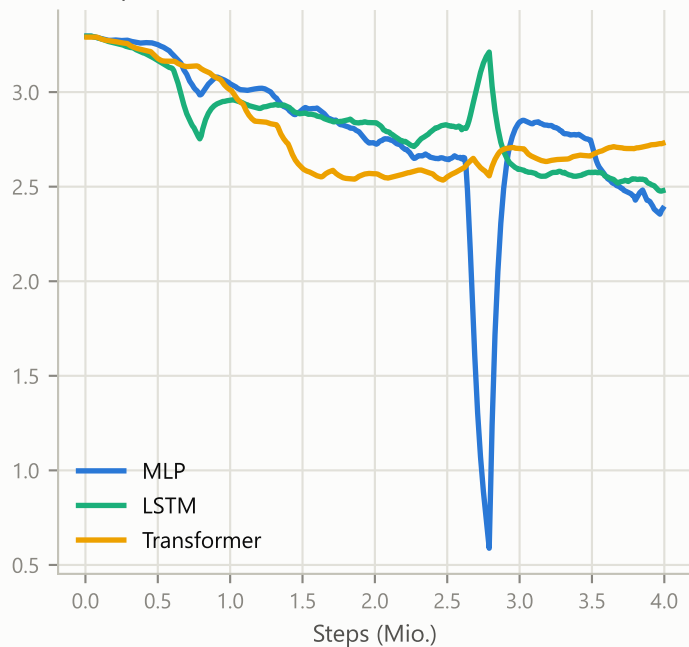
Entropie
