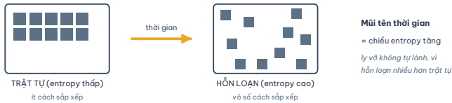
Hình 2.1 · Mũi tên thời gian – vũ trụ trôi từ trật tự sang hỗn loạn đơn giản vì có vô số cách để lộn xộn hơn là gọn gàng
