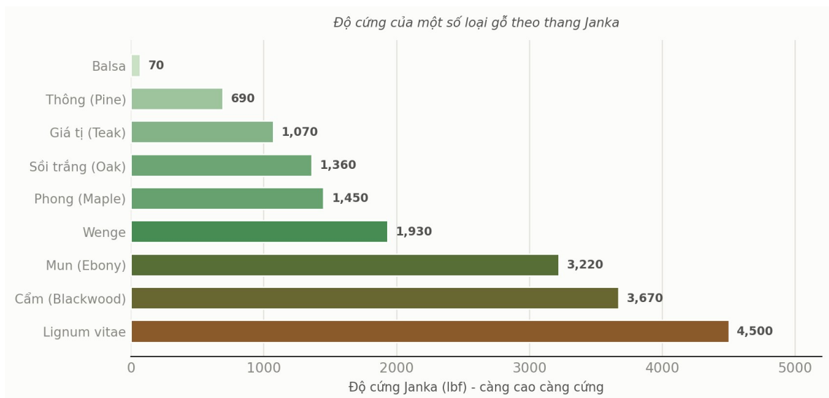
Hình 4. Độ cứng của một số loại gỗ theo thang Janka (đơn vị lbf): từ gỗ balsa siêu nhẹ, qua thông, giá tị, sồi, đến những loại cứng nhất như gỗ mun, cẩm và lignum vitae
