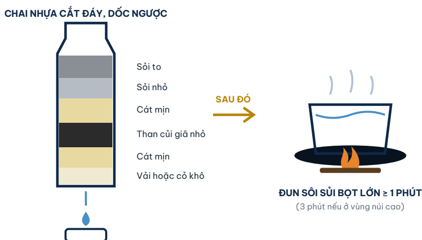
Hình 2.1 – Bộ lọc nước tự chế từ chai nhựa và bước khử trùng bằng đun sôi: lọc trước, đun sau
