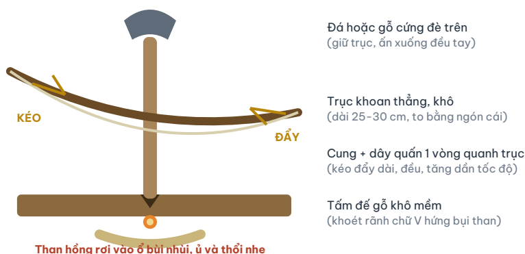
Hình 3.1 – Cấu tạo bộ cung khoan lửa: kỹ thuật tạo lửa bằng ma sát kinh điển của nhân loại
