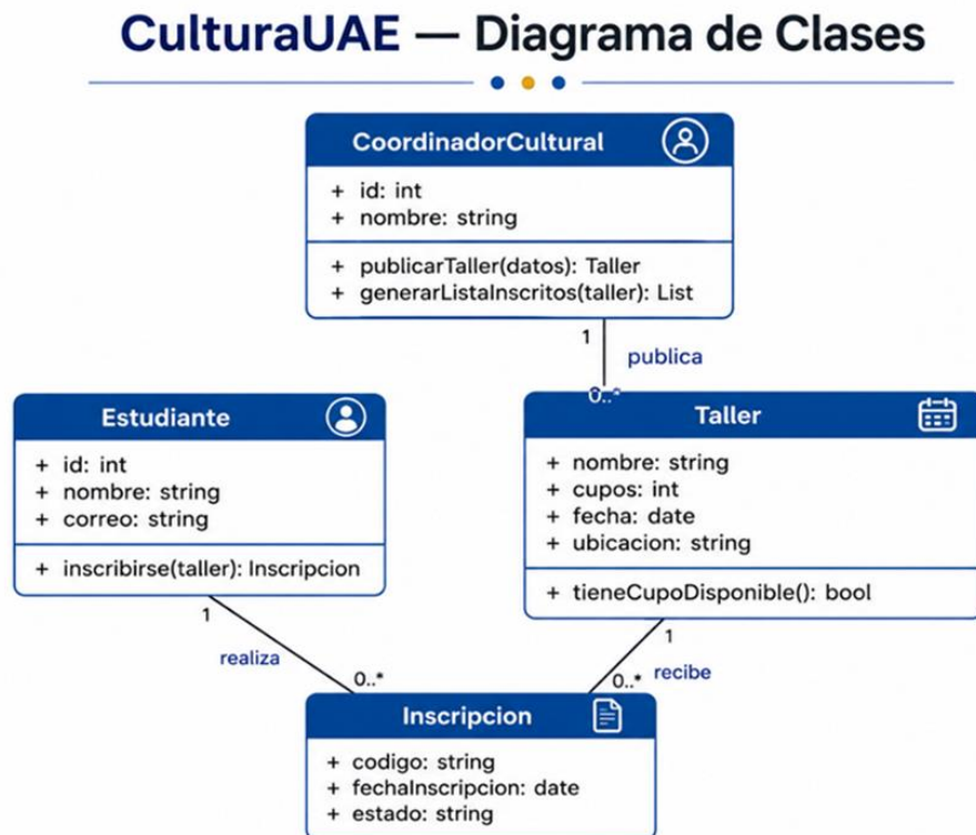
Figura 2. Diagrama de clases de CulturaUAE.
