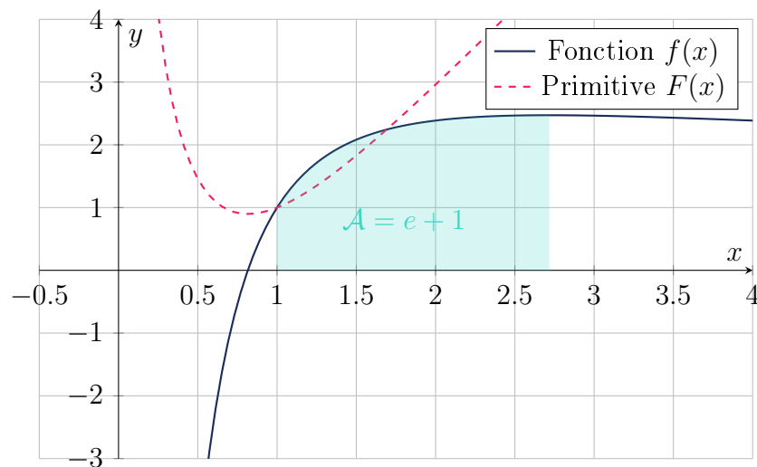
Courbes de la fonction f et de sa primitive F
