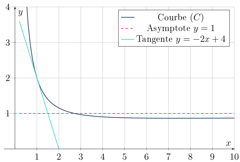
Courbe (C) et Asymptotes
