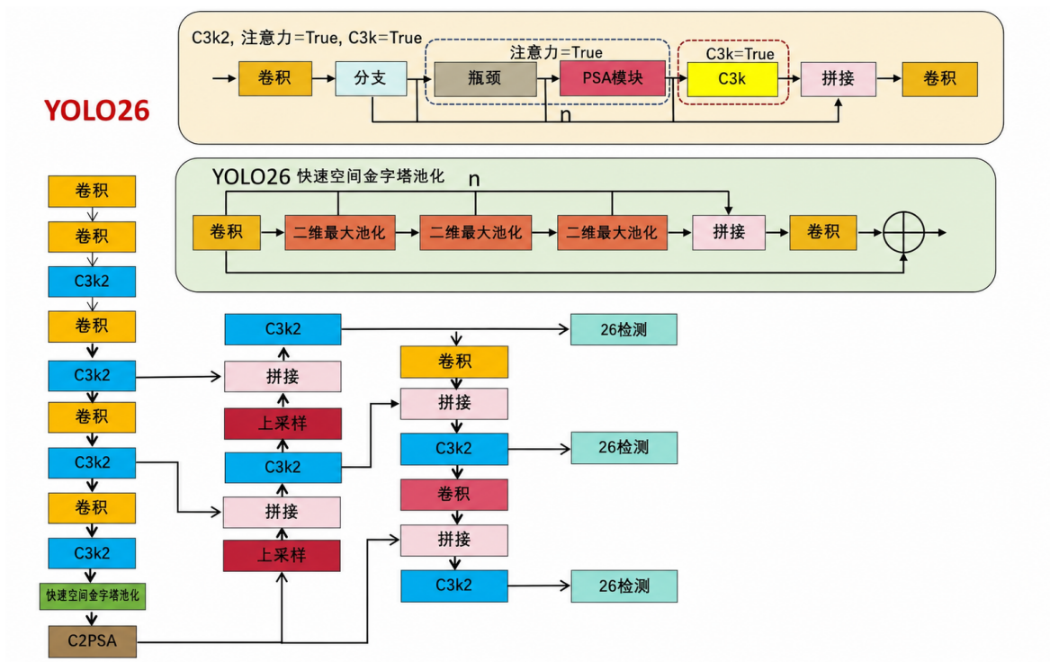
图 3.8 YOLO26 网络结构图，引自 [19]
