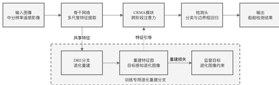
图 3.3 DRENet 方法示意
