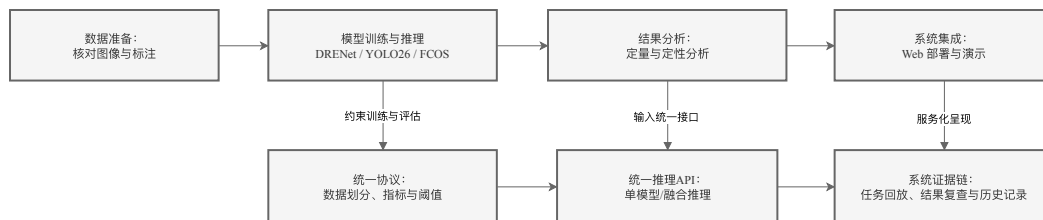
图 1.1 技术路线图
