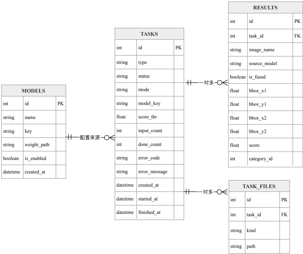
图 5.2 系统数据库 ER 图
