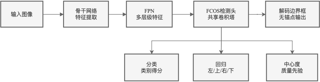
图 3.4 FCOS 检测流程示意
