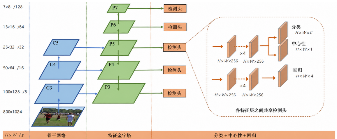
图 3.6 FCOS 网络结构图（基于文献 [4] 图示翻译整理）
