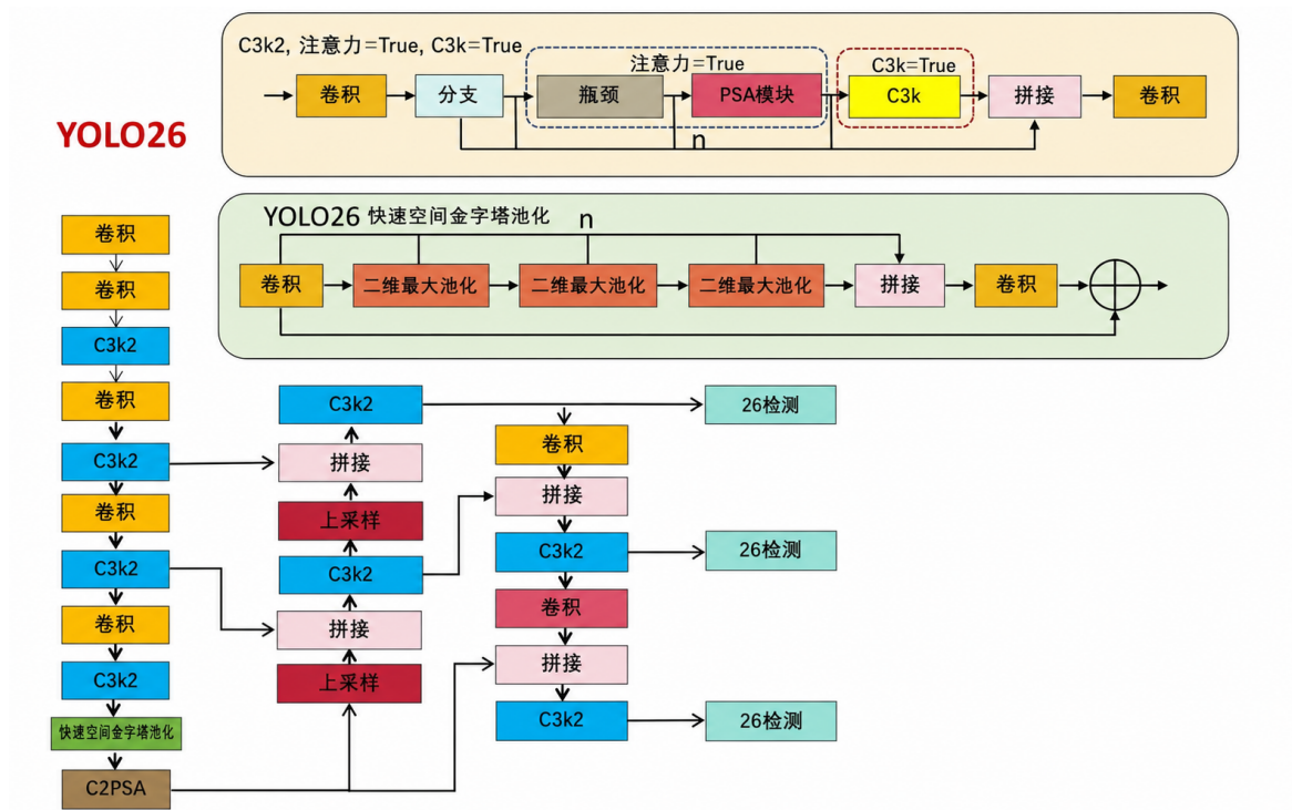
图 3.8 YOLO26 网络结构图
