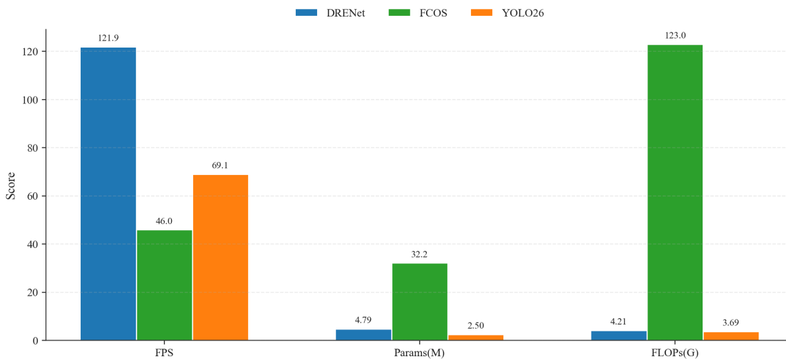
图 4.2 三模型效率与复杂度对比柱状图
