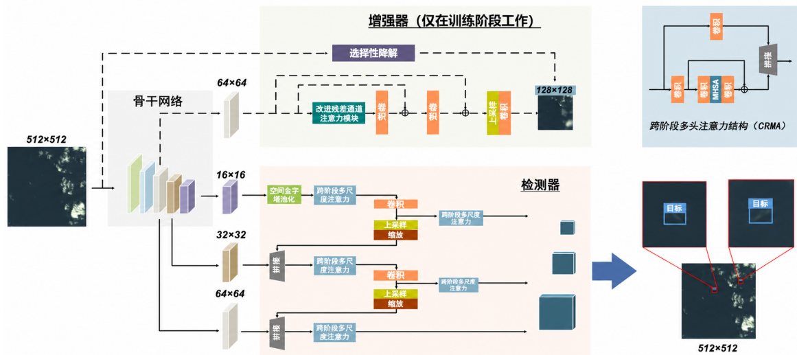
图 3.4 DRENet 网络结构图（基于文献 [17] 图示翻译整理）
