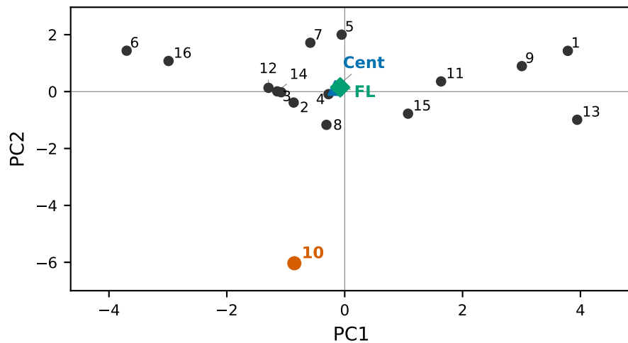
L2
