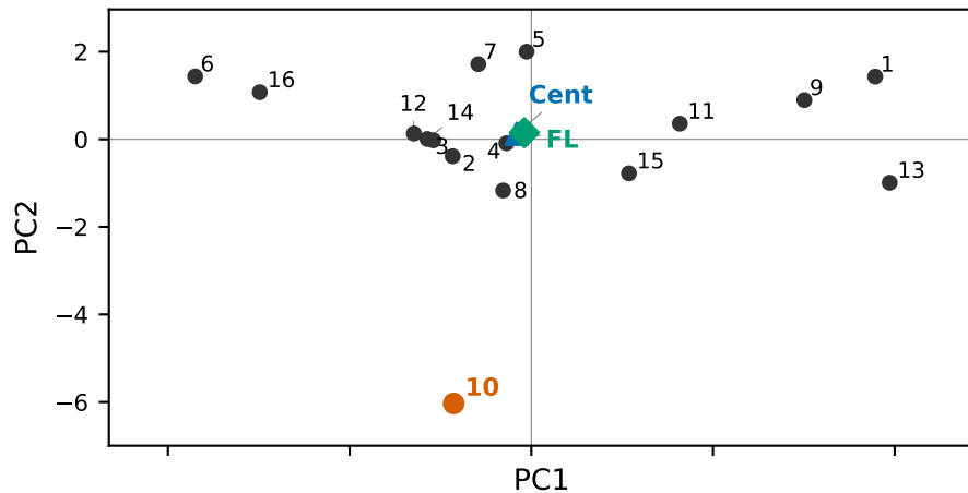
L2
