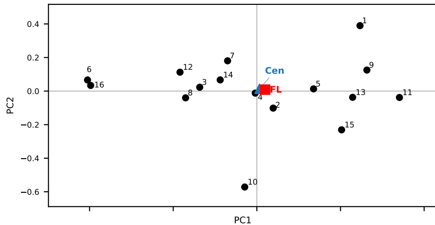
L2
