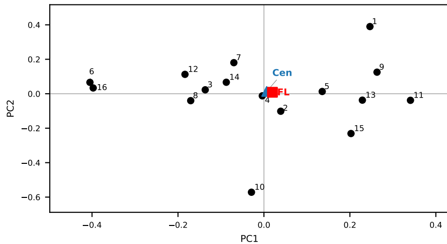
L2
