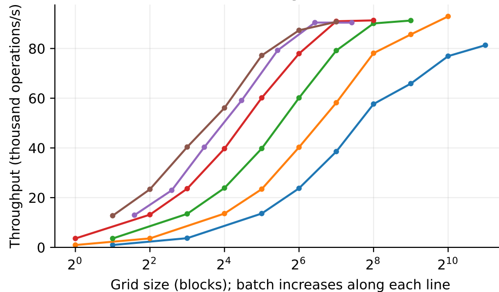
Encaps
