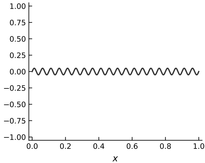
wiggle: \|\cdot\|_\infty = 0.05 , \|\cdot\|_{L^2} = 0.035
