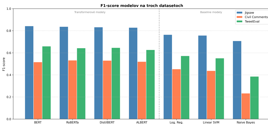
Obrázok 4–2 F1-score transformerových a baseline modelov na troch datasetoch: Jigsaw (trénovací), Civil Comments a TweetEval
