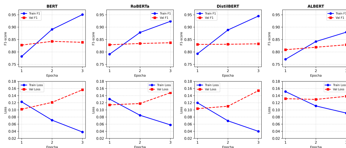
Obrázok 4–1 Priebek tréovania transformerových modelov: F1-score (hore) a Loss (dole) na tréningovej a validačnej množine počas troch epoch
