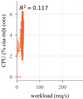
RCAEval (benchmark)
