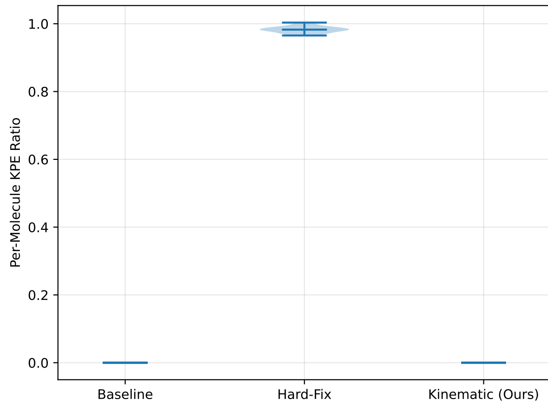
(d) Per-Molecule KPE Ratio Distribution (N=50)
