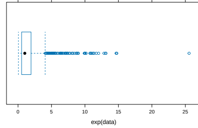
(d) Boxplot
