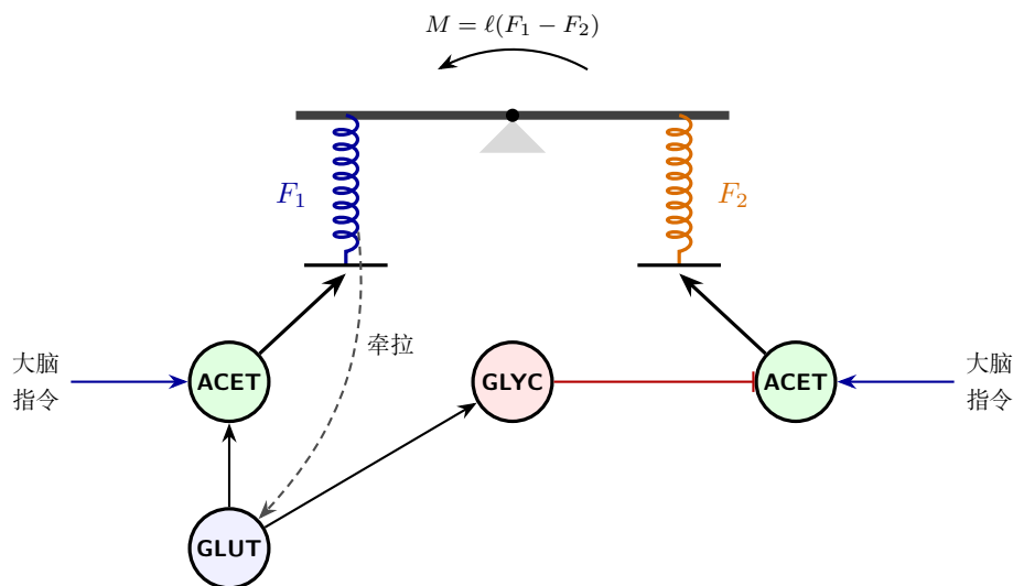
图 13.2: 一个关节上的两块肌肉和最快的反馈环路。 ACET 神经元接收大脑的指令，把关节拉向不同方向；力之差使关节转动，力之和使它更僵硬。左侧肌肉的牵拉传感器（ GLUT ）兴奋该肌肉自己的 ACET 神经元，并经 GLYC 中间神经元抑制拮抗肌的神经元——即第 3 章的否决。
