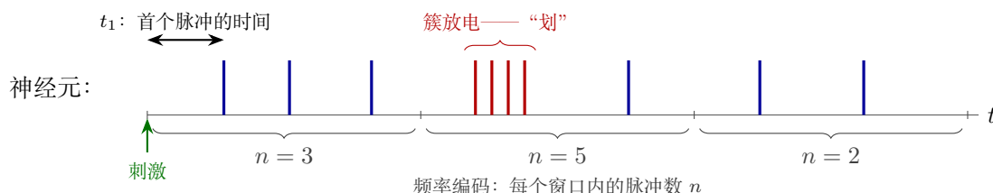
图 4.1: 摩尔斯电码与神经元的电码。同一串脉冲可以有不同读法：数出每 50 ms 窗口内的脉冲数 (4.4 节)，测量延迟 t_1 (4.4)，或者注意到簇放电——“划” (4.7)。
