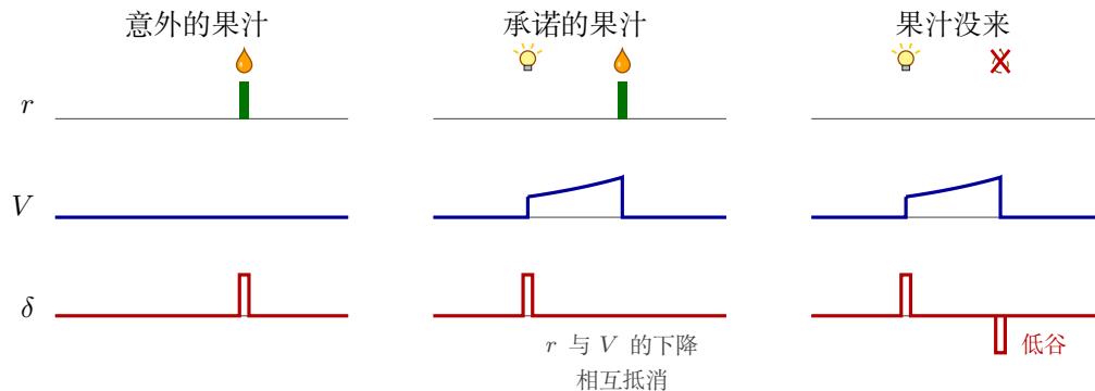
图 6.4: 误差 (6.8) 的三种情况; 自上而下依次为奖励 r 、期望 V 和误差 \delta 。左: 没有期望, 果汁完全出乎意料。中: 灯使 V 跃升, 这是 dV/dt 的跃变, \delta 的爆发落在灯亮时。之后 V 恰好按视野的要求增长, \delta = 0 ; 果汁到来时, 奖励 r 与 V 的下降相互抵消。右: V 在没有奖励时下降——低谷。这就是图 1.4 中的爆发、转移和低谷, 只是现在能看出它们从何而来。
