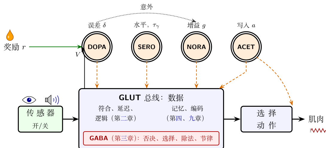
图 10.1: 整台机器。 GLUT 总线把数据从传感器送到动作选择; GABA 控制总线内部的数据流。双线圆圈是广播通道; 虚线箭头表示把它们的信号发给整个网络, 每条通道有自己的旋钮。 DOPA 接收奖励 r 和来自总线内部评论器的预期 V (第 六 章); 点线箭头是一个假说: NORA 通过异常大的误差得知意外 (第 八 章)。
