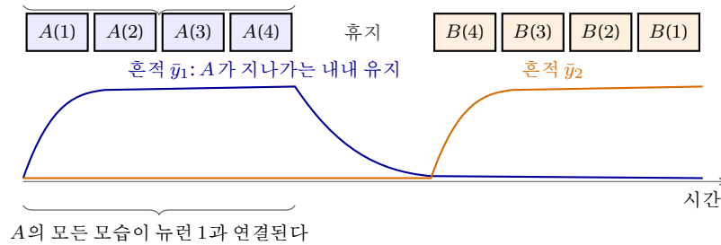
그림 12.2: 영상이 불변성을 가르치는 방식, 도식. 물체 A 가 네 위치를 지나가고, 휴지가 있는 뒤 물체 B 가 온다. A 의 첫 모습에서 이긴 뉴런의 혼적 (12.2)은 지나가는 내내 유지되어, A 의 모든 모습이 한 뉴런과 연결된다. 휴지가 혼적을 지우므로 B 는 다른 뉴런에게 간다.
