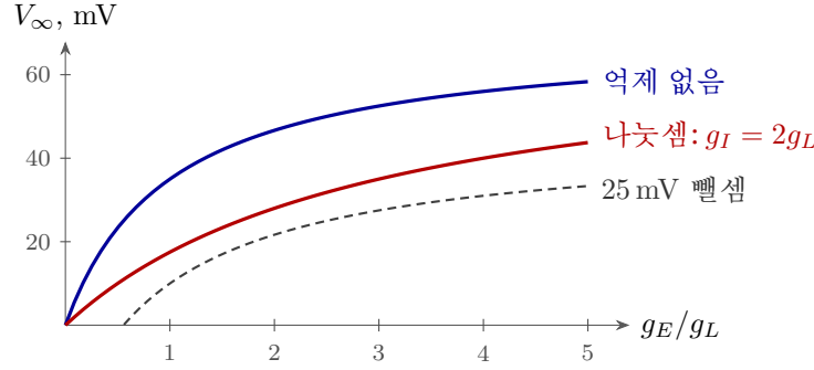
그림 3.2: 분로 억제는 전압에서 빼지 않고 전압을 나눈다. 파란 곡선은 억제가 없을 때의 정상 상태 전압 (3.3), 빨간 곡선은 억제성 컨덕턴스 g_I = 2g_L 이 있을 때이다. 빨간 곡선은 파란 곡선을 가로로 세 배 늘린 것과 같다. 입력을 1 + g_I/g_L = 3 으로 나눈 샘이다. 파선은 일정한 25 mV를 빼는 억제이다. 곡선 전체가 내려갈 뿐 기울기는 변하지 않는다.
