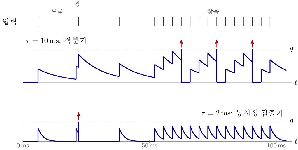
그림 4.3: 같은 입력, 서로 다른 두 수신자. 스파이크마다 전압이 w 만큼 올랐다가 뉴런 모델 (2.1)에 서처럼 흘러내린다. 빨간 화살표는 수신자의 스파이크이다. 느린 수신자( \tau = 10 \text{ ms} , \theta = 2.5w )는 스파이크가 많은 곳에서 발화하고 쌍은 알아채지 못한다. 빠른 수신자( \tau = 2 \text{ ms} , \theta = 1.5w )는 창 (2.2) 안의 쌍에만 발화하고, 맞지만 일치하지 않는 흐름은 흘려보낸다.
