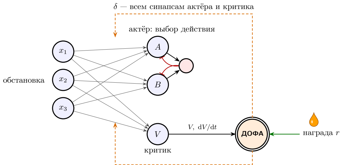
Рис. 6.5: Сеть, которая учится выбирать действия. Серые стрелки — ГЛУТ -синапсы с меняющимися весами; красный кружок — ГАМК -нейрон; двойной кружок — ДОФА -ритмоводитель, вычисляющий \delta по (6.8); штриховые стрелки — широковещательная рассылка \delta .
