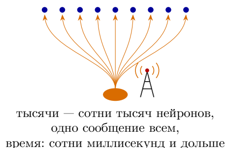
Рис. 1.3: Два способа передачи. Слева — адресная шина, похожая на почту с адресом на конверте; красным выделен один нейрон и два его получателя. Справа — широковещательная, как радиостанция: небольшая группа нейронов-источников, и одно и то же сообщение получают все.
