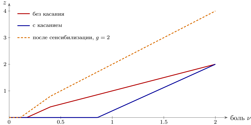
Рис. 14.2: Выход ворот (14.2) в зависимости от силы боли. Касание поднимает порог и приглушает слабую и среднюю боль, но не сильную. Сенситализация (штриховая линия) вдвое увеличивает усиление: та же боль передаётся вдвое громче, а порог опускается.
