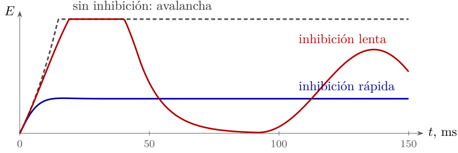
Figura 3.4: Frecuencia de un grupo GLUT con realimentación w_{EE} = 1.5 , \tau_E = 10 ms, tras conectar la entrada. Sin inhibición (discontinua), la actividad crece sin límite. Con una inhibición de fuerza w_{EI}w_{IE} = 2 y \tau_I = 2 ms (curva azul), se estabiliza en el nivel E^* = h/(1 - 1.5 + 2) = 0.67h . Con la misma inhibición, pero lenta, \tau_I = 30 ms (curva roja), la actividad oscila.
