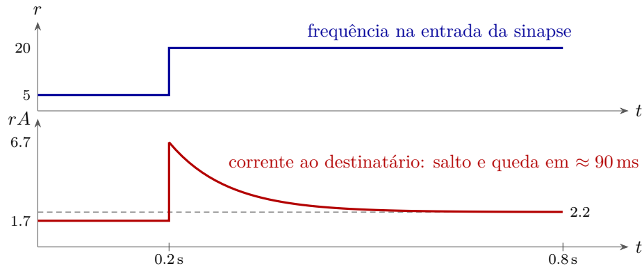
Figura 4.4: Sinapse com depressão pela fórmula (4.6), com U = 0.5 , \tau_{\text{rec}} = 0.8 s; corrente em unidades de A_0 por segundo; a linha tracejada é a corrente de regime: ela subiu só de 1.7 para 2.2, e no instante do salto, até 6.7. A sinapse informa ao destinatário que a frequência mudou, não qual ela é.
