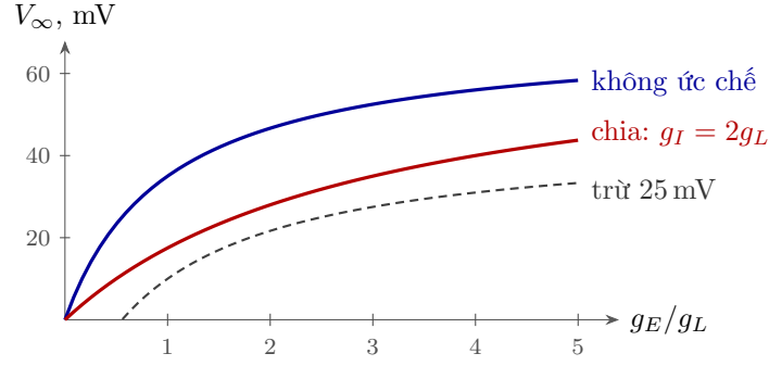
Hình 3.2: Ức chế sun chia điện áp chứ không trừ khỏi nó. Đường xanh là điện áp xác lập (3.3) khi không có ức chế, đường đỏ là khi có độ dẫn ức chế g_I = 2g_L . Đường đỏ chính là đường xanh bị kéo giãn gấp ba theo chiều ngang: như thể đầu vào bị chia cho 1 + g_I/g_L = 3 . Đường nét đứt là ức chế trừ đi một lượng không đổi 25 mV: cả đường cong hạ xuống, độ dốc không đổi.
