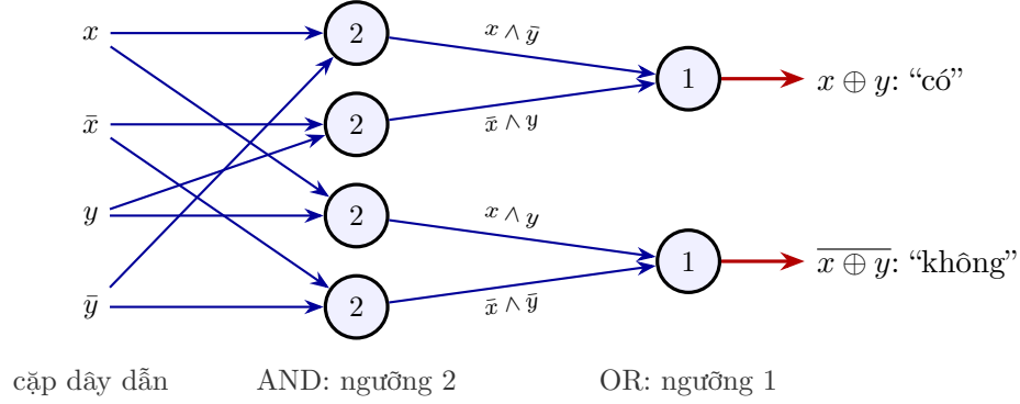
Hình 2.2: XOR trên mã hai dây, chỉ gồm các nơ-ron GLUT . Số trong vòng tròn là ngưỡng, tính theo đơn vị trọng số của một đầu vào. Bốn nơ-ron AND nhận ra bốn tổ hợp đầu vào, hai nơ-ron OR gom chúng thành cặp dây kết quả.
