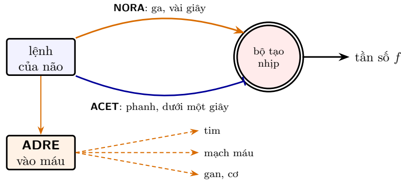
Hình 16.1: Hai dây dẫn trái dấu tới bộ tạo nhịp tim: ga NORA chậm, phanh ACET nhanh. Phía dưới là cũng chân ga ấy nhưng đi qua bus quảng bá: các tế bào ADRE thả adrenaline vào máu, và mọi cơ quan có thụ thể phù hợp đều nhận được tín hiệu (mũi tên nét đứt).
