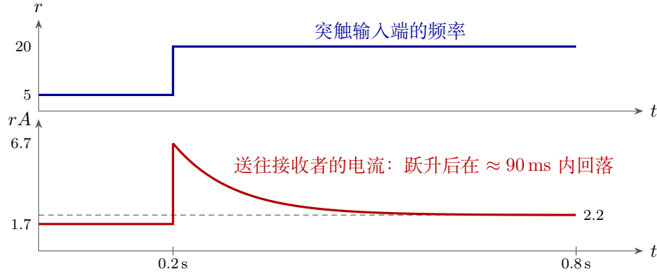
图 4.4: 按公式 (4.6) 工作的压抑型突触, U = 0.5 , \tau_{\text{rec}} = 0.8 \text{ s} ; 电流以每秒 A_0 为单位, 虚线是稳态电流: 它只从 1.7 升到 2.2, 而在跃变瞬间达到 6.7。突触告诉接收者的是频率变了, 而不是频率是多少。
