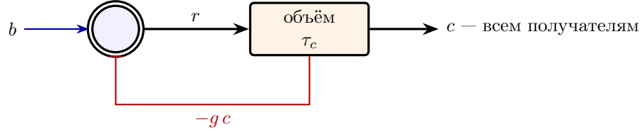
Рис. 5.2: SERO -нейрон с обратной связью через собственный медиатор: концентрация c идёт ко всем получателям и тормозит сам нейрон. В модели это регулятор уровня; в мозге такая роль петли — гипотеза.
