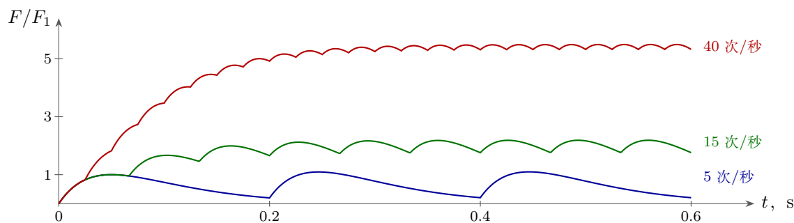
图 13.1: 肌肉作为数模转换器：一个运动单位规则发放时的力 (13.2)， T_c = 50 ms。稀疏的脉冲产生分离的抽搐，密集的脉冲融合成平稳的力——正如图 5.3 中密集的脉冲融合成平稳的浓度。
