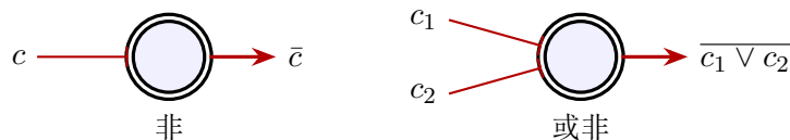
图 5.1: 由 SERO 神经元构成的逻辑。双圆圈是起搏器：在平稳的背景输入下它自己工作，直到被抑制。带横杠的线是抑制性受体， s = -1 ； c 、 c_1 、 c_2 是接收者周围各体积中的血清素浓度。左为“非”，右为“或非”。
