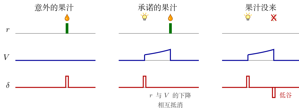
图 6.4: 误差 (6.8) 的三种情况; 自上而下依次为奖励 r 、期望 V 和误差 \delta 。左: 没有期望, 果汁完全出乎意料。中: 灯使 V 跃升, 这是 dV/dt 的跃变, \delta 的尖峰落在灯亮时。之后 V 恰好按视野的要求增长, \delta = 0 ; 果汁到来时, 奖励 r 与 V 的下降相互抵消。右: V 在没有奖励时下降——低谷。这就是图 1.4 中的尖峰、转移和低谷, 只是现在能看出它们从何而来。
