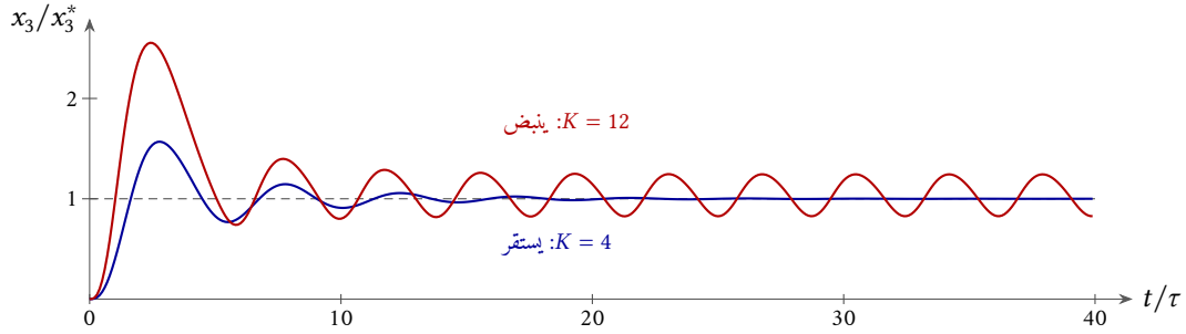
شكل 16.2: سلسلة من ثلاث مراحل بتغذية راجعة وفق (16.2)؛ مستوى الهرمون الأخير بوصفه كسراً من قيمة التوازن x_3^* . حين يكون كسب الحلقة أقل من ثمانية يستقر المستوى؛ وحين يزيد عليها تولّد السلسلة بنفسها نبضات منتظمة.
