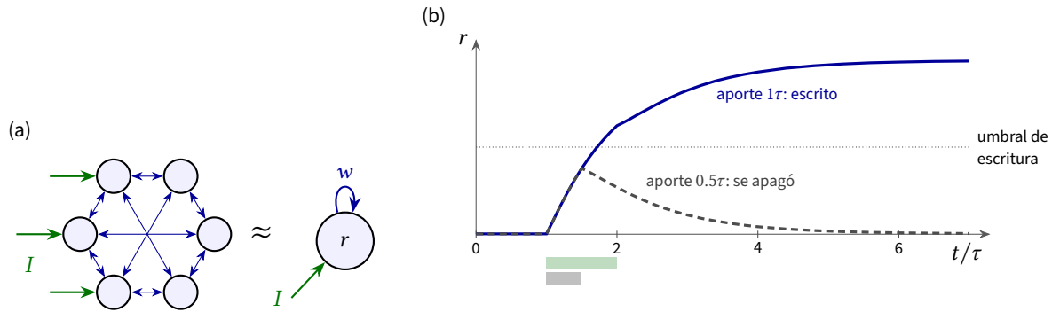
Figura 2.4: Un grupo fuertemente conectado consigo mismo. (a) Muchas neuronas GLUT que se excitan entre sí se comportan como una sola neurona de frecuencia r que se excita a sí misma con fuerza w ; desde fuera llega el aporte I . (b) Frecuencia del grupo en el tiempo con w = 1 y la misma curva f que en la fig. 2.5. El aporte I = 0.6 se aplica durante el tiempo marcado por la franja bajo el eje. Si dura 1\tau , el grupo alcanza a cruzar el punto inestable r = 0.5 , se enciende y sigue encendido cuando el aporte termina. Si dura solo 0.5\tau , no llega a ese punto y vuelve a apagarse: para escribir un bit, el aporte debe durar más de aproximadamente 0.7\tau .
