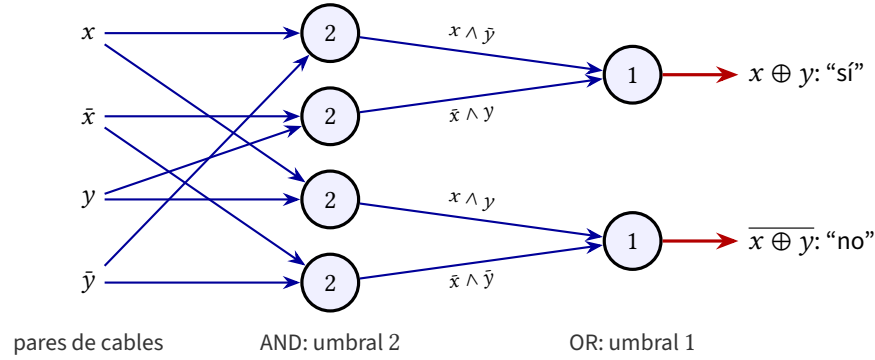
Figura 2.2: OR exclusivo en código de dos cables, solo con neuronas GLUT. El número del círculo es el umbral en unidades del peso de una entrada. Cuatro neuronas AND reconocen las cuatro combinaciones de entradas, y dos neuronas OR las reúnen en el par de cables de la respuesta.
