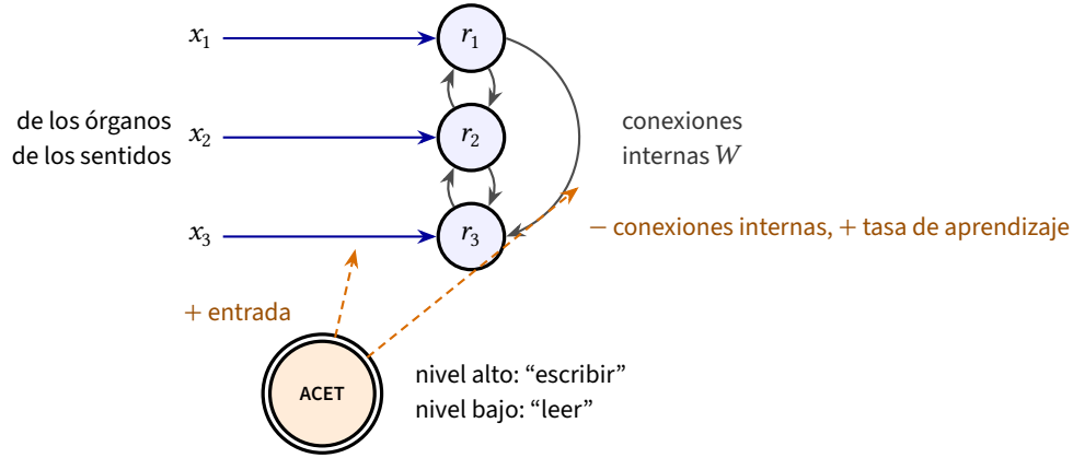
Figura 9.1: ACET como línea de habilitación de escritura. Las neuronas r_i reciben la entrada x_i de los órganos de los sentidos (flechas azules) y se excitan entre sí a través de las conexiones internas W (grises), en las que se guardan los patrones. La acetilcolina (flechas discontinuas) refuerza la entrada, debilita las conexiones internas y facilita el cambio de los pesos, como en (9.1).
