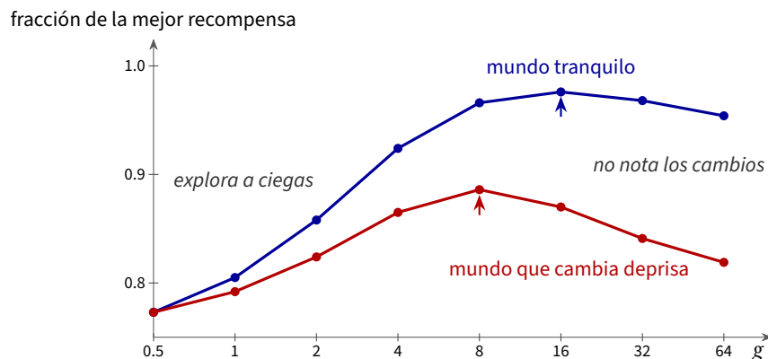
Figura 8.3: Fracción de la mejor recompensa posible con ganancia g constante (escala logarítmica en g ). Curva azul: el mundo cambia en promedio una vez cada mil intentos; roja: una vez cada veinte. Las flechas marcan la mejor g : en el mundo que cambia deprisa es la mitad. Promedio de 60 ejecuciones de 4000 intentos.
