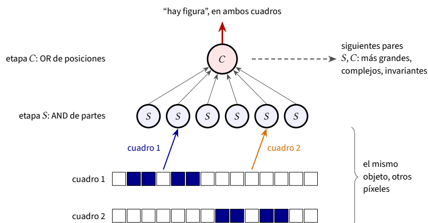
Figura 12.1: Un par de etapas de la cadena. Las neuronas S buscan la misma combinación de partes en distintos lugares; la neurona C responde si la encontró en cualquier sitio (12.1). La figura del cuadro 1 y la del cuadro 2 excitan neuronas S distintas, pero la misma C . Los siguientes pares de etapas repiten lo mismo con combinaciones cada vez más grandes y complejas.
