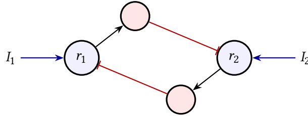
Figura 3.3: Elección entre dos. Dos grupos de neuronas GLUT (azules) se inhiben mutuamente a través de intermediarios GABA (rojos).
