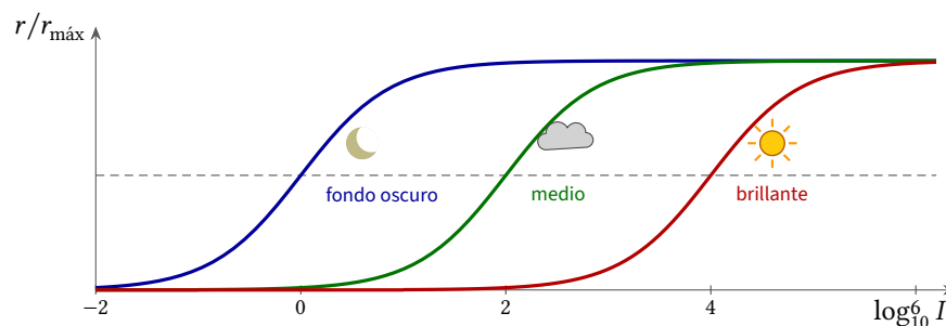
Figura 11.2: Control de ganancia del sensor de luz según (11.2). Cada curva abarca dos o tres órdenes de brillo; al pasar a un fondo más brillante, \sigma crece y la curva se desplaza por el eje logarítmico. Juntas, las curvas desplazadas cubren todo el rango.
