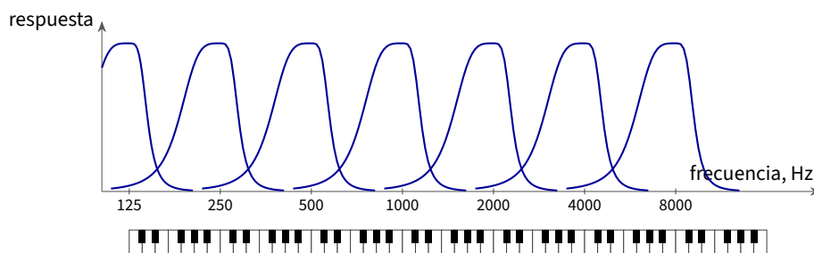
Figura 11.3: El oído como banco de filtros pasa banda, esquema. Cada curva es la respuesta de los sensores de un tramo a sonidos de distinta frecuencia; las frecuencias centrales van de octava en octava, como las teclas en una escala logarítmica. Los filtros reales tienen una pendiente de alta frecuencia abrupta y una de baja frecuencia suave. Abajo, un teclado: en él, como en el oído, a cada octava le toca el mismo espacio.
