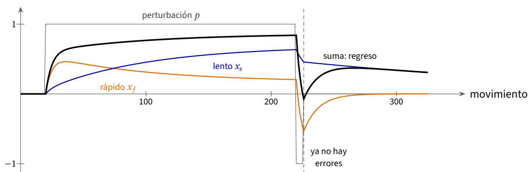
Figura 15.2: Dos procesos de aprendizaje según el modelo (15.3), A_f = 0.92 , B_f = 0.1 , A_s = 0.996 , B_s = 0.02 . Doscientos movimientos con la perturbación p = 1 y luego seis con la inversa, p = -1 , hasta que la suma vuelve a cero. Tras la línea discontinua dejan de llegar errores, y la suma vuelve sola a la corrección anterior: el proceso rápido olvidó la perturbación inversa; el lento recuerda la directa.
