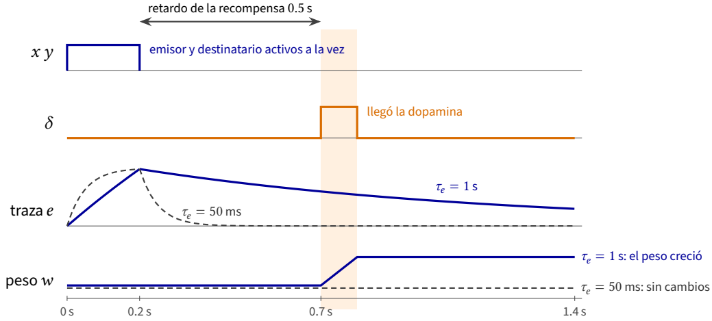
Figura 6.2: Trazas según la regla (6.5). La actividad conjunta dura 0.2 s; la dopamina llega medio segundo después de que termina. Las trazas se muestran en fracciones de su máximo. La traza lenta ( \tau_e = 1 s) sigue viva en ese momento; la rápida ( \tau_e = 50 ms) se desvaneció hace tiempo.
