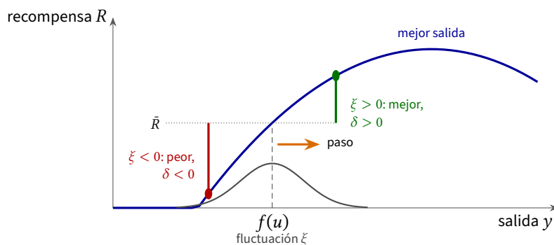
Figura 6.3: El ruido como búsqueda (6.6). La salida de la neurona fluctúa alrededor de f(u) . Una desviación aleatoria a la derecha (verde) dio más de lo esperado, \delta > 0 ; a la izquierda (roja), menos, \delta < 0 . En ambos casos el producto \delta \xi es positivo, y el peso se desplaza a la derecha, hacia donde crece la recompensa. En promedio, el paso es proporcional a la pendiente R' : en la cima de la colina las desviaciones a ambos lados son igual de malas, y los pasos se anulan.
