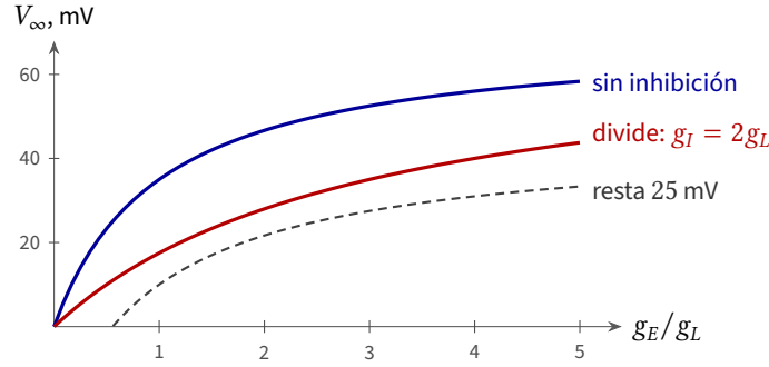
Figura 3.2: La inhibición de derivación divide el voltaje, no le resta. La curva azul es el voltaje estacionario (3.3) sin inhibición; la roja, con conductancia inhibidora g_I = 2g_L . La roja es la misma azul estirada tres veces en horizontal: como si la entrada se dividiera por 1 + g_I/g_L = 3 . La discontinua es una inhibición que resta 25 mV constantes: la curva baja entera y la pendiente no cambia.
