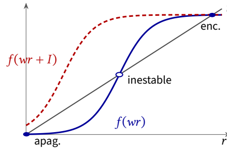
Figura 2.5: Memoria a partir de un grupo de neuronas GLUT con realimentación fuerte. La curva continua, sin aporte externo: dos cortes estables con la recta r , “apagado” y “encendido”, y uno inestable entre ellos. Un aporte breve I (curva discontinua) deja solo el superior.
