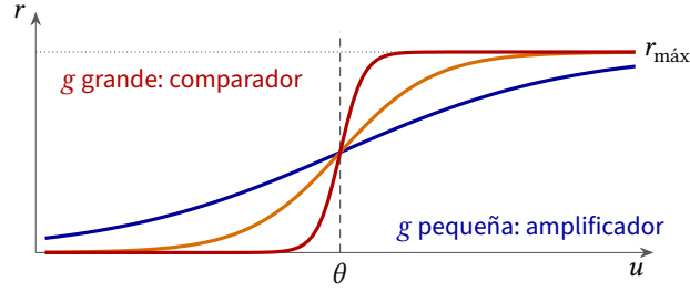
Figura 8.1: La característica de transferencia (8.1) con tres valores de la ganancia g .
