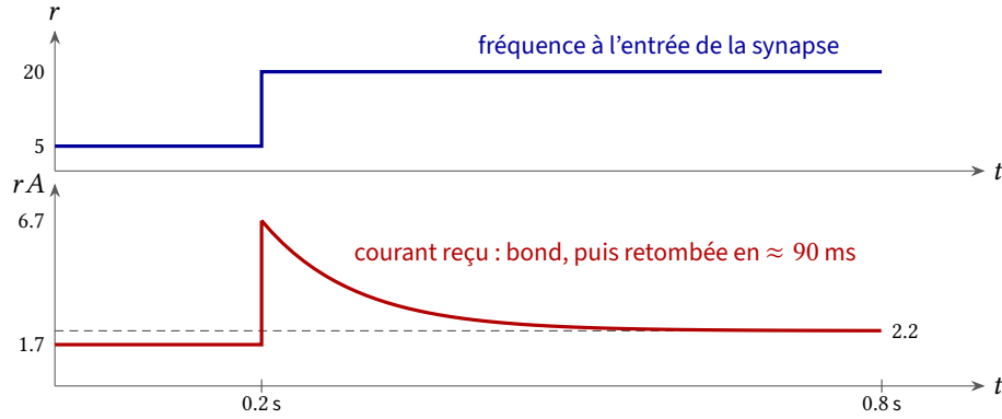
FIGURE 4.4 : Synapse à dépression d'après la formule (4.6), pour U = 0.5 , \tau_{\text{rec}} = 0.8 s; courant en unités de A_0 par seconde; en tirets, le courant établi : il n'est passé que de 1.7 à 2.2, mais a bondi à 6.7 au moment du saut. La synapse informe le destinataire que la fréquence a changé, non de sa valeur.
