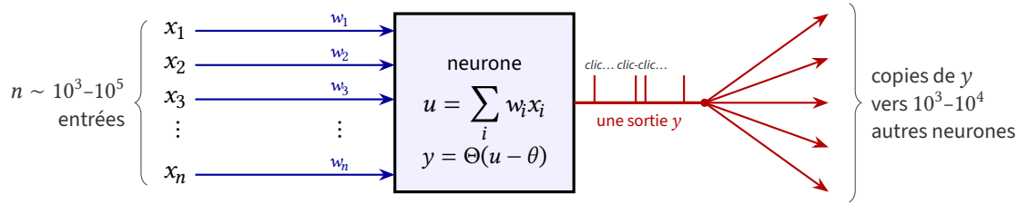
FIGURE 1.1 : Le neurone vu par un ingénieur. De nombreuses entrées x_i , chacune avec son poids w_i ; à l'intérieur, une somme pondérée u et une comparaison au seuil \theta ( \Theta est la fonction échelon : 1 si l'argument est positif, 0 sinon); une seule sortie y , une suite d'impulsions démultipliée par ramification vers des milliers de destinataires.
