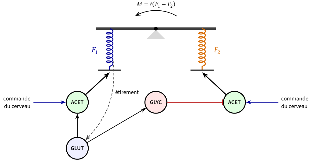
FIGURE 13.2 : Deux muscles pour une articulation et la boucle de rétroaction la plus rapide. Les neurones ACET reçoivent les commandes du cerveau et tirent l'articulation dans des sens opposés; la différence des forces la fait tourner, leur somme la rend plus raide. Le capteur d'étirement ( GLUT ) du muscle de gauche excite son propre neurone ACET et, par un intermédiaire GLYC , inhibe le neurone du muscle antagoniste : le veto du chapitre 3.
