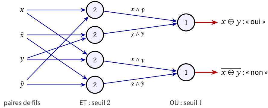
FIGURE 2.2 : OU exclusif en code à deux fils, avec des neurones GLUT seulement. Le nombre dans le cercle est le seuil, en unités du poids d'une entrée. Quatre neurones ET reconnaissent les quatre combinaisons d'entrées, deux neurones OU les rassemblent en une paire de fils de réponse.
