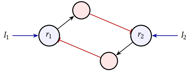
FIGURE 3.3 : Choisir entre deux. Deux groupes de neurones GLUT (en bleu) s'inhibent mutuellement par des intermédiaires GABA (en rouge).
