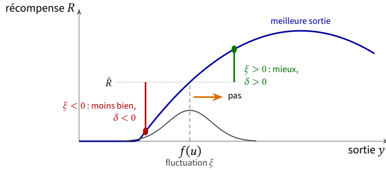
FIGURE 6.3 : Le bruit comme recherche (6.6). La sortie du neurone fluctue autour de f(u) . Un écart aléatoire vers la droite (en vert) a rapporté plus que prévu, \delta > 0 ; vers la gauche (en rouge), moins, \delta < 0 . Dans les deux cas, le produit \delta \xi est positif, et le poids se déplace vers la droite, là où la récompense croît. En moyenne, le pas est proportionnel à la pente R' : au sommet de la colline, les écarts des deux côtés sont également mauvais, et les pas s'annulent.
