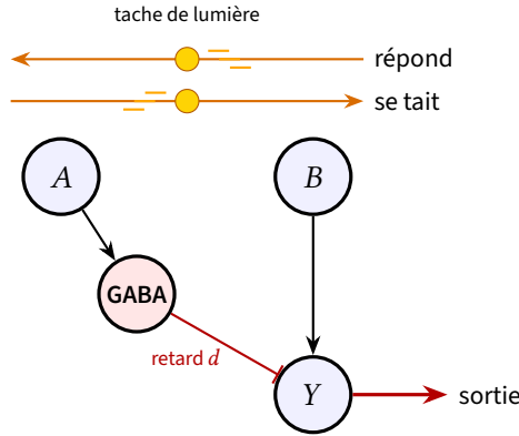
FIGURE 3.1 : Détecteur de direction du mouvement. B excite Y , A l'inhibe par un intermédiaire GABA avec un retard d . Pour un mouvement de A vers B à une vitesse proche de \Delta x/d , l'inhibition éteint l'excitation; pour le mouvement inverse, elle arrive trop tard. La tache jaune avec ses traits est la lumière qui court au-dessus des capteurs.
