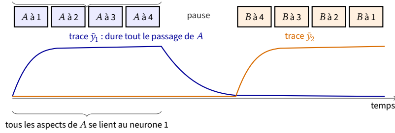
FIGURE 12.2 : Comment la vidéo enseigne l'invariance, schéma. L'objet A passe par quatre positions, puis vient une pause, puis l'objet B . La trace (12.2) du neurone qui a gagné sur le premier aspect de A dure tout le passage, et tous les aspects de A se retrouvent liés à un seul neurone. La pause efface la trace, et B revient à un autre neurone.
