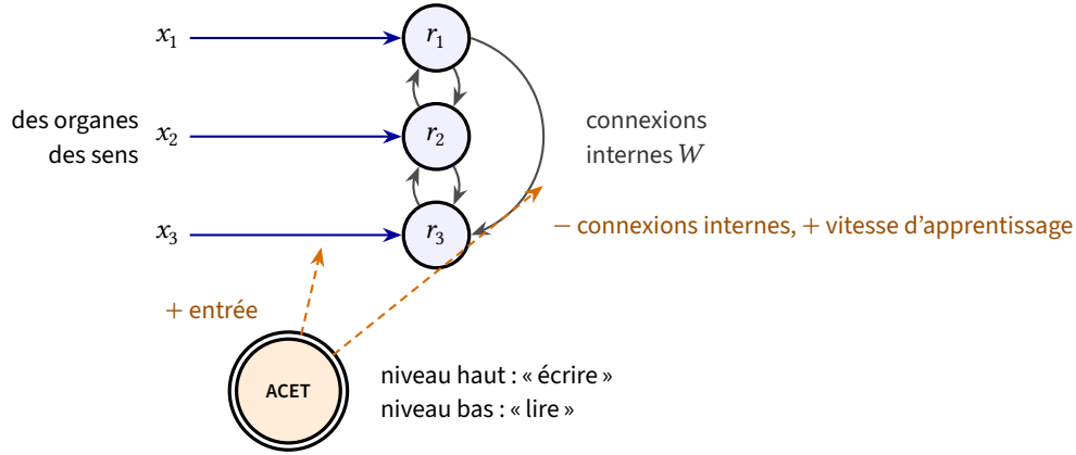
FIGURE 9.1 : ACET comme ligne de validation d'écriture. Les neurones r_i reçoivent l'entrée x_i des organes des sens (flèches bleues) et s'excitent mutuellement par les connexions internes W (en gris), qui stockent les motifs. L'acétylcholine (flèches en tirets) renforce l'entrée, affaiblit les connexions internes et facilite la modification des poids, comme dans (9.1).
