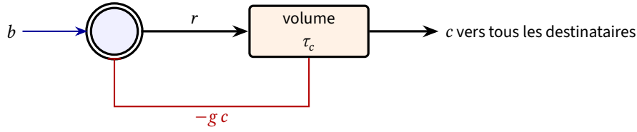
FIGURE 5.2 : Neurone SERO rétrocontrôlé par son propre neurotransmetteur : la concentration c va à tous les destinataires et inhibe le neurone lui-même. Dans le modèle, c est un régulateur de niveau ; dans le cerveau, ce rôle de la boucle est une hypothèse.
