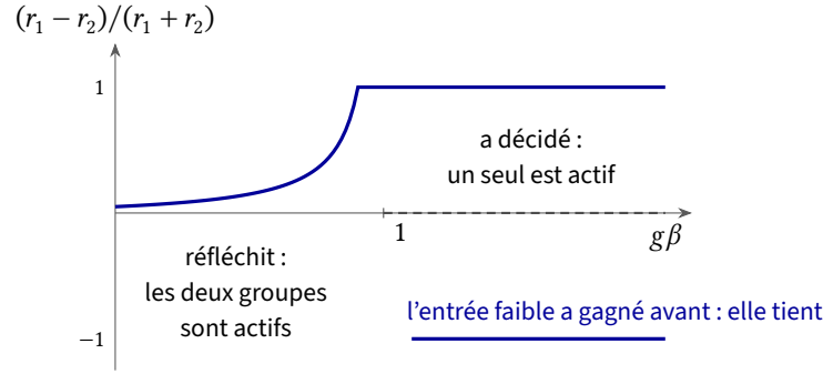
FIGURE 8.2 : Choix entre deux options pour différents gains ; les entrées diffèrent de \varepsilon = 0.05 . Pour g\beta > 1 , les deux décisions sont stables (traits pleins) ; la victoire de l'entrée faible pour g\beta > (1 + \varepsilon)/(1 - \varepsilon) \approx 1.1 , et le réseau maintient celle qu'il a déjà prise ; l'état symétrique (en tirets) est instable.
