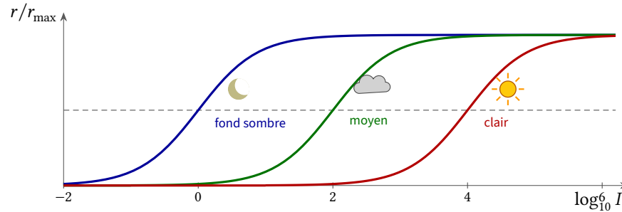
FIGURE 11.2 : Réglage du gain d'un capteur de lumière selon (11.2). Chaque courbe couvre deux ou trois ordres de grandeur de luminosité; quand on passe à un fond plus clair, \sigma augmente et la courbe glisse le long de l'axe logarithmique. Ensemble, les courbes glissantes couvrent toute la plage.
