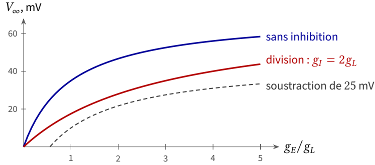
FIGURE 3.2 : L'inhibition shuntante divise la tension au lieu d'en soustraire. Courbe bleue : tension établie (3.3) sans inhibition ; courbe rouge : avec une conductance inhibitrice g_I = 2g_L . La rouge est la même que la bleue, étirée trois fois à l'horizontale : tout se passe comme si l'entrée était divisée par 1 + g_I/g_L = 3 . En tirets : une inhibition qui soustrait 25 mV constants ; la courbe descend en bloc, sa pente ne change pas.
