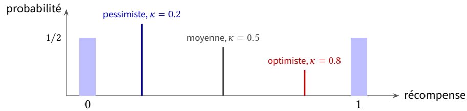
FIGURE 7.1 : La distribution de la récompense enregistrée par un ensemble de neurones DOPA . Récompense 0 ou 1 avec la probabilité 1/2 (barres bleues); un neurone de fraction \kappa aboutit à l'estimation V = \kappa (7.2).
