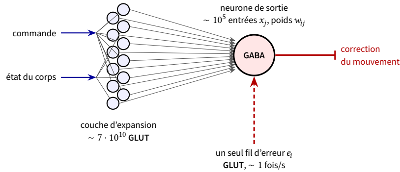
FIGURE 15.1 : Le circuit d'apprentissage supervisé, tel que le cerveau semble le réaliser. La commande et l'état du corps sont décomposés par une immense couche de neurones GLUT en un long vecteur x_j ; le neurone GABA de sortie en fait la somme avec les poids w_{ij} . Un unique fil d'erreur apporte e_i ; la coïncidence de l'erreur avec une entrée active affaiblit le poids de cette entrée, comme dans la règle (15.1).
