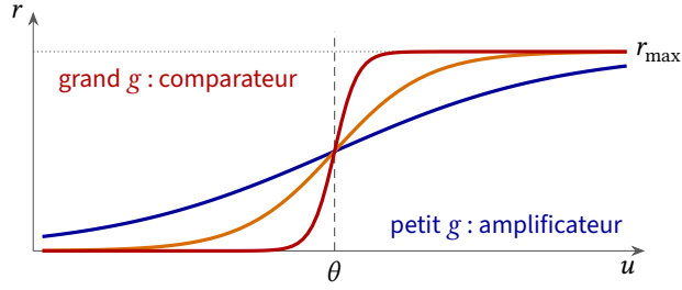
FIGURE 8.1 : La caractéristique de transfert (8.1) pour trois valeurs du gain g .
