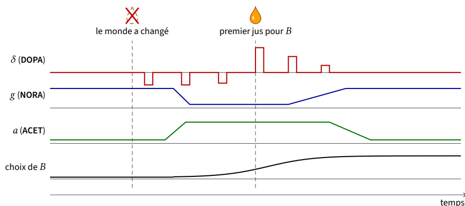
FIGURE 10.2 : Un seul événement suivi à travers toute la machine. C'est un schéma qualitatif fondé sur les modèles et les hypothèses des chapitres 6–9, non le résultat d'un calcul. Après le changement, DOPA répond par des creux; les creux répétés font monter, par hypothèse, le signal de surprise, NORA baisse le gain, ACET active l'écriture; le premier jus pour B donne une bouffée, le choix passe à B , et les boutons reviennent à leur place.
