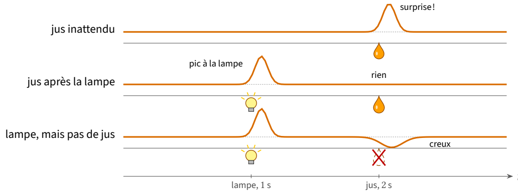
FIGURE 1.4 : Fréquence des impulsions des neurones DOPA dans trois expériences (schéma d'après [2]). Le pointillé est la fréquence de fond, constante. La lampe est le signal, la goutte est le jus, la goutte barrée est un jus promis mais non donné. La réponse est l'erreur de prédiction (1.2).
