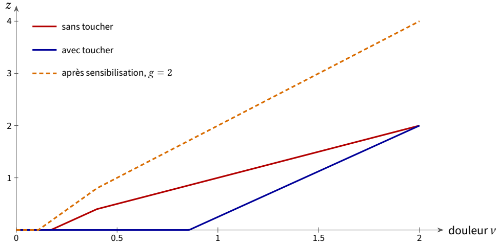
FIGURE 14.2 : Sortie du portillon (14.2) en fonction de l'intensité de la douleur. Le toucher relève le seuil et atténue la douleur faible et moyenne, mais pas la douleur forte. La sensibilisation (trait en tirets) double le gain : la même douleur est transmise deux fois plus fort, et le seuil s'abaisse.
