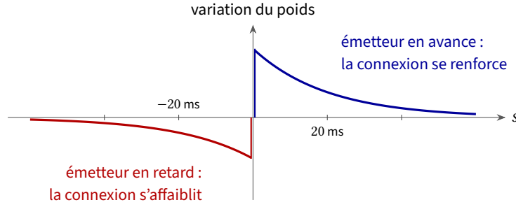
FIGURE 6.1 : La règle de Hebb temporelle. En abscisse, s = t_{\text{dest}} - t_{\text{ém}} , le retard de l'impulsion du destinataire sur celle de l'émetteur; \tau_{\pm} = 20 ms, A_- = 0.6A_+ . La fenêtre, large de quelques dizaines de millisecondes, est du même ordre que la fenêtre de coïncidence (2.2).
