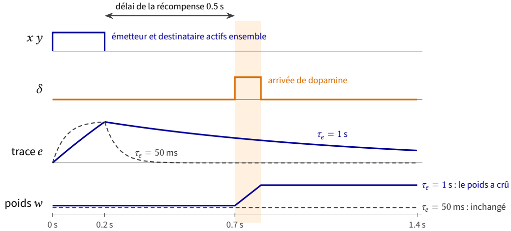
FIGURE 6.2 : La trace selon la règle (6.5). L'activité conjointe dure 0.2 s ; la dopamine arrive une demi-seconde après sa fin. Les traces sont représentées en fraction de leur maximum. La trace lente ( \tau_e = 1 s) est encore vivante à ce moment, la trace rapide ( \tau_e = 50 ms) s'est effacée depuis longtemps.
