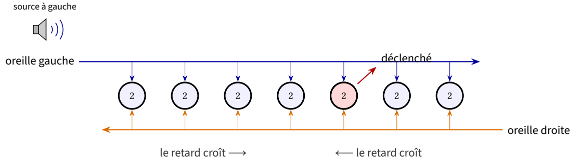
FIGURE 2.3 : Déterminer la direction d'un son. Les signaux des deux oreilles courent l'un vers l'autre; chaque cercle est un détecteur de coïncidences de seuil 2. Si le son arrive plus tard à l'oreille droite, les signaux se rencontrent à droite du milieu, selon la formule (2.5). La sortie du réseau est le numéro du neurone déclenché. Ici la source est à gauche : le son est arrivé plus tôt à l'oreille gauche.
