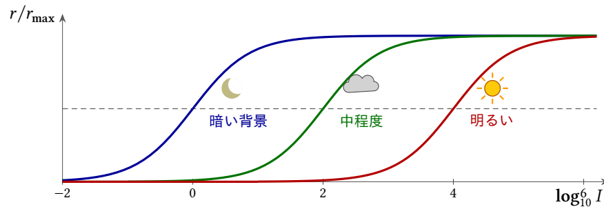
図 11.2: (11.2) による光センサのゲイン調整。各曲線は明るさの2～3桁をカバーする。より明るい背景に移ると \sigma が大きくなり、曲線は対数軸に沿ってずれる。ずれていく曲線全体でレンジ全体をカバーする。
