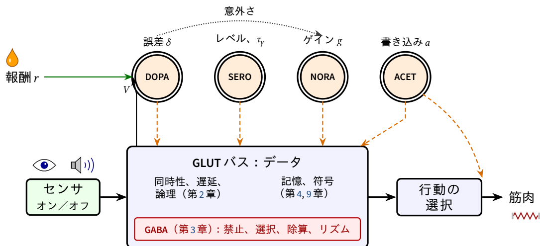
図 10.1: マシンの全体像。GLUT バスはデータをセンサから行動の選択へ運び、GABA がその内部の流れを制御する。二重丸はブロードキャストチャンネル、破線の矢印はその信号を網全体へ配ることを表し、チャンネルごとに自分のつまみがある。DOPA は報酬 r と、バス内部の評価器（クリティック）からの期待値 V を受け取る（第 6 章）。点線の矢印は、NORA が異常に大きな誤差から意外さを知るという仮説を表す（第 8 章）。
