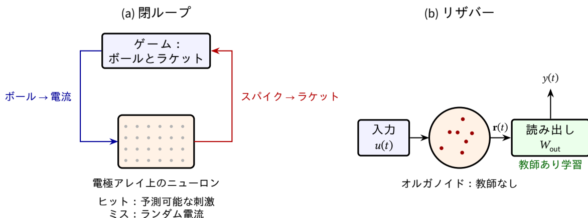
図 21.1: 生きたネットワークに計算させる二つの方法。(a) 閉ループ：ボールの位置は電流として与えられ、運動領域のスパイクがラケットを動かし、打った後の予測可能な刺激またはランダムな刺激が教師となる。(b) リザバー (21.2)：オルガノイドには学習信号を与えない。オルガノイドは入力をもつ多数の非線形応答に分解する。誤差から学習するのは外側の線形読み出し一つだけである。ただしオルガノイド自身の結合もこのとき変化する。教師なしで。
