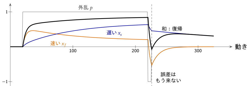
図 15.2: モデル (15.3) による二つの学習過程、 A_f = 0.92, B_f = 0.1, A_s = 0.996, B_s = 0.02 。外乱 p = 1 で 200 回の動き、次に和がゼロに戻るまで逆向きの p = -1 で 6 回。破線の後には誤差が届かなくなり、和はひとりで古い補正へ戻る。速い過程は逆向きの外乱を忘れ、遅い過程は順向きの外乱を覚えている。
