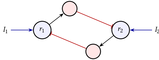
図 3.3: 二者択一。GLUT ニューロンの二つの群（青）が、GABA の仲介役（赤）を通じて互いに抑制し合う。
