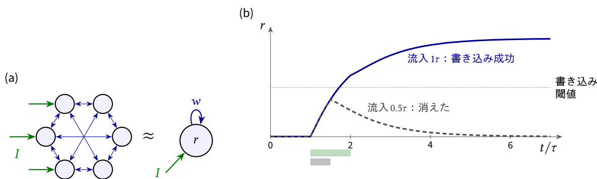
図 2.4: 自分自身と強く結合した群。(a) 互いに興奮させ合う多数の GLUT ニューロンは、強さ w で自分自身を興奮させる発火率 r の 1 個のニューロンのようにふるまう。外部からは流入 I が来る。(b) w = 1 、図 2.5 と同じ曲線 f のときの群の発火率の時間変化。流入 I = 0.6 は、軸の下で示した時間だけ与えられる。流入が 1\tau 続けば、群は不安定点 r = 0.5 を越え、燃え上がり、流入が終わっても燃え続ける。 0.5\tau だけなら、この点まで届かず消えて元に戻る。ビットを書き込むには、流入はおおよそ 0.7\tau より長く続かなければならない。
