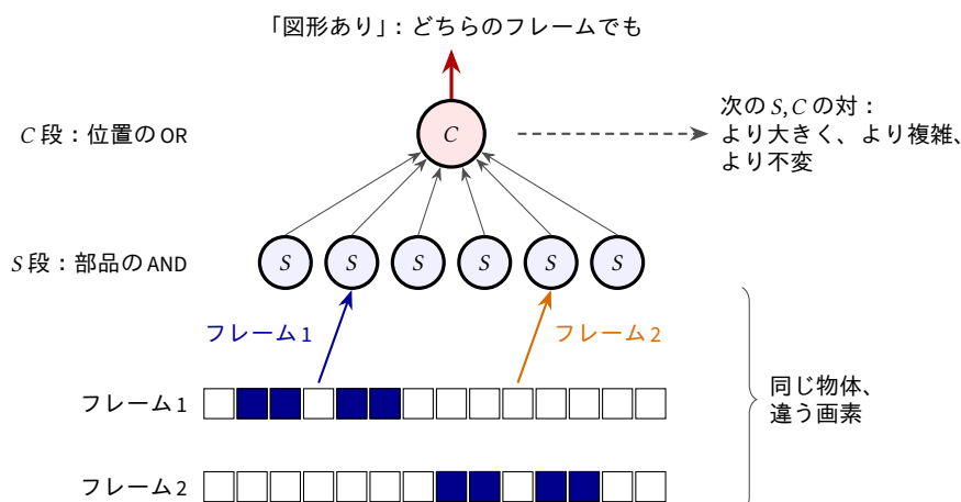
図 12.1: パイプラインの一对の段。S ニューロンは同じ部品の組み合わせを異なる場所で探し、C ニューロンはそれがどこかで見つければ応答する (12.1)。フレーム1とフレーム2の図形は異なる S ニューロンを興奮させるが、同じ C を興奮させる。次の段の対は、同じことをより大きく複雑な組み合わせについて繰り返す。
