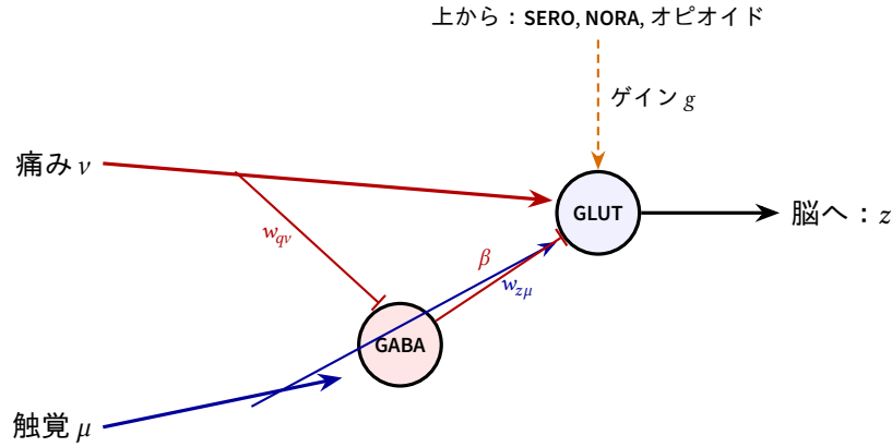
図 14.1: モデル(14.2)による脊髄の痛みのゲート。出力 GLUT ニューロンは痛み v と、触覚 \mu からの弱い興奮を受ける。抑制性の介在ニューロン (GABA または GLYC) は触覚で興奮し、ゲート理論の仮定では痛みでオフになる。上からはブロードキャストチャンネルを通じてゲイン g が来る。
