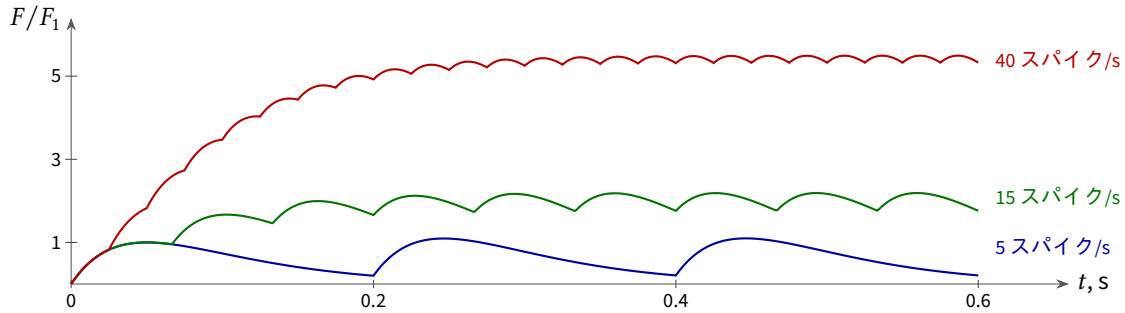
図 13.1: D/A 変換器としての筋肉：1 個の運動単位の規則的なスパイクに対する力 (13.2)、 T_c = 50 ms。まばらなスパイクは個々の単収縮を生み、頻繁なスパイクは融合して平らな力になる。図 5.3 で頻繁なスパイクが融合して平らな濃度になったのと同じである。
