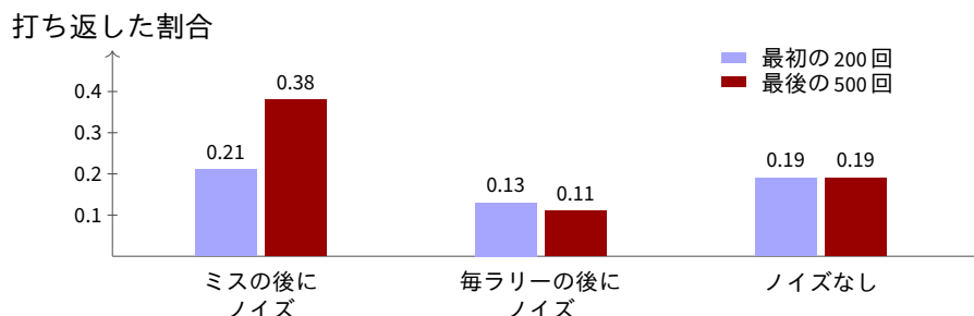
図 22.2: 「ミスでかき混ぜる」モデル (dishbrain_model.py): 2000 ラリーの最初と最後で打ち返した割合。40 個のモデル培養の平均。学習が進むのは、揺さぶりがミスの後に来てヒットの後には来ないときだけである。セッション内の有意な伸びが完全なフィードバックのときだけだった実験と同じである。
