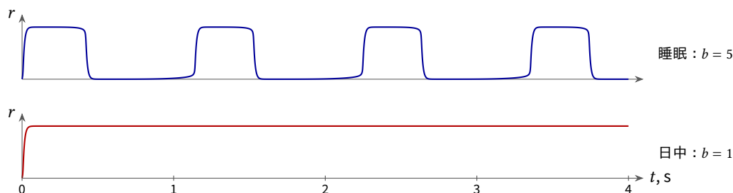
図 20.2: 二つのモードにおける同じ群 (20.2) : w = 5 、 I = 2 、 \theta = 2.5 、 \tau = 10 \text{ ms} 、 \tau_a = 0.3 \text{ s} 。疲労が強いと ( b = 5 、ノンレム睡眠のように)、群は周期 1.1 s で活動と静止の間を振動する (モデルの値。皮質では周期は 1 秒より長く、麻酔下では約 3 s)。疲労を弱めると ( b = 1 、アセチルコリンの作用がこれにあたる)、同じ群が一様に働く。
