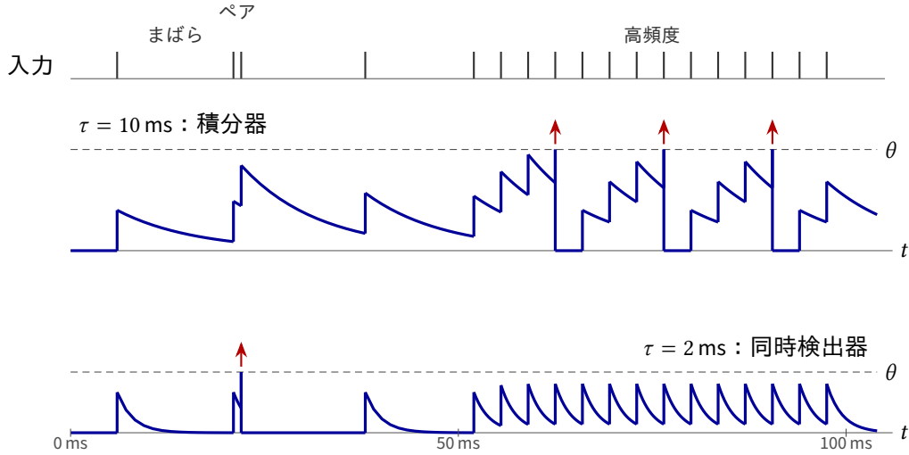
図 4.3: 同じ入力と二つの異なる受け手。各スパイクは電圧を w だけ上げ、その後はニューロンのモデル (2.1) のように電圧が流れ落ちる。赤い矢印は受け手のスパイクである。遅い受け手 ( \tau = 10 ms、 \theta = 2.5w ) はスパイクが多いところで発火し、ペアには気づかない。速い受け手 ( \tau = 2 ms、 \theta = 1.5w ) は窓 (2.2) の中のペアにだけ発火し、高頻度でも同時でない列は見逃す。
