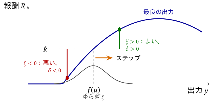
図 6.3: 探索としてのノイズ (6.6)。ニューロンの出力は f(u) のまわりでゆらぐ。右へのランダムなずれ (緑) は期待より多くを得て \delta > 0 、左へのずれ (赤) は少なく \delta < 0 。どちらの場合も積 \delta\xi は正で、重みは報酬が増える右へ動く。平均するとステップは傾き R' に比例する。山の頂上では両側へのずれが同じように悪く、ステップは打ち消し合う。
