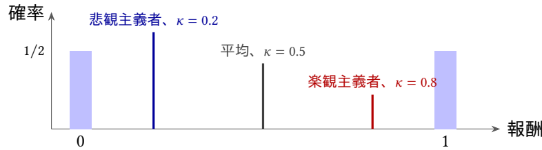
図 7.1: DOPA ニューロンの集まりに記録された報酬の分布。報酬は確率 1/2 で 0 または 1 (青い棒)。割合 \kappa のニューロンは推定値 V = \kappa に至る (7.2)。
