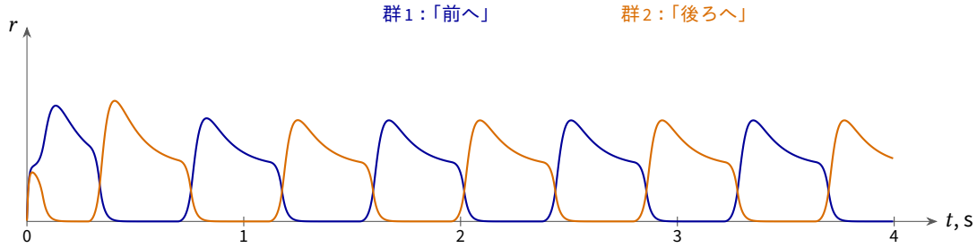
図 13.3: モデル (13.6) によるリズム発生器 : I = 1, \beta = 2, b = 2, \tau = 20 \text{ ms}, \tau_a = 0.4 \text{ s} . 相互抑制と疲労を持つ二つの群は、入力が一定の信号であるにもかかわらず、周期 0.84 \text{ s} で交代に働く。
