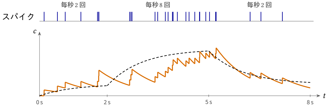
図 5.3: スパイクからレベルへ。上は SERO ニューロンのスパイク。2秒間はまばら、3秒間は密、その後ふたたびまばらになる。下は \tau_c = 1\text{s} のときのセロトニン濃度 (5.3)。破線はスパイクが完全に等間隔だった場合の同じ量。
