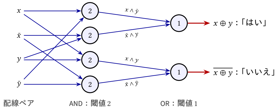
図 2.2: 2 線式符号による排他的 OR。GLUT ニューロンだけで作る。丸の中の数、入力 1 本の重みを単位とした閾値である。4 個の AND ニューロンが入力の 4 通りの組み合わせを認識し、2 個の OR ニューロンがそれを答えの配線ペアにまとめる。
