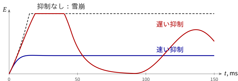
図 3.4: 入力オンにした後の、帰還 w_{EE} = 1.5 、 \tau_E = 10 ms をもつ GLUT 群の発火率。抑制がないと（破線）活動は際限なく増える。強さ w_{EI}w_{IE} = 2 、 \tau_I = 2 ms の抑制があると（青の曲線）、活動はレベル E^* = h/(1 - 1.5 + 2) = 0.67h に落ち着く。同じ強さでも遅い抑制 \tau_I = 30 ms では（赤の曲線）、活動は振動する。
