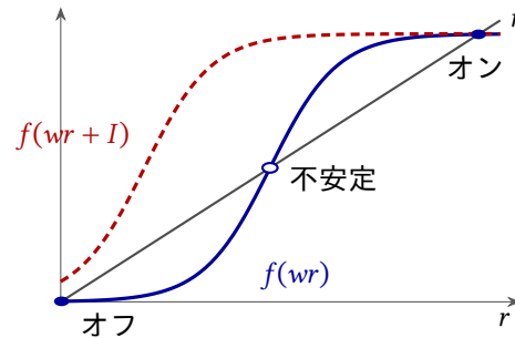
図 2.5: 強い帰還をもつ GLUT ニューロン群によるメモリ。実線は外部流入がない場合で、直線 r との安定な交点が二つ（「オフ」と「オン」）、その間に不安定な交点が一つある。短い流入 I （破線）があると、上の交点だけが残る。
