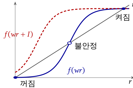
그림 2.5: 되먹임이 강한 GLUT 뉴런 무리로 만든 메모리. 실선 곡선은 바깥 유입이 없을 때이다. 직선 r 과 안정한 교점 둘, 즉 “꺼짐”과 “켜짐”이 있고, 그 사이에 불안정한 교점이 있다. 짧은 유입 I (파선 곡선)가 가해지면 위쪽 교점만 남는다.
