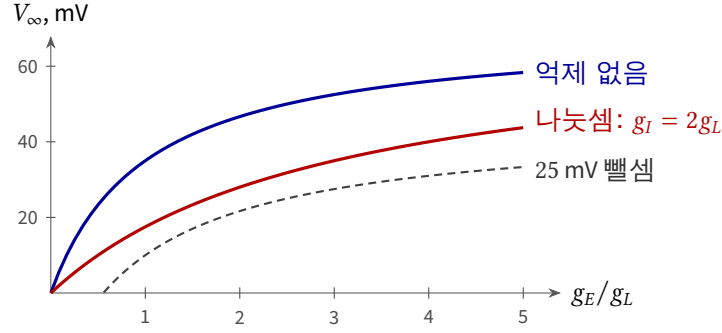
그림 3.2: 분로 억제는 전압에서 빠지 않고 전압을 나눈다. 파란 곡선은 억제가 없을 때의 정상 상태 전압 (3.3), 빨간 곡선은 억제성 컨덕턴스 g_I = 2g_L 이 있을 때이다. 빨간 곡선은 파란 곡선을 가로로 세 배 늘린 것과 같다. 입력을 1 + g_I/g_L = 3 으로 나눈 셈이다. 파선은 일정한 25 mV를 빼는 억제이다. 곡선 전체가 내려갈 뿐 기울기는 변하지 않는다.
