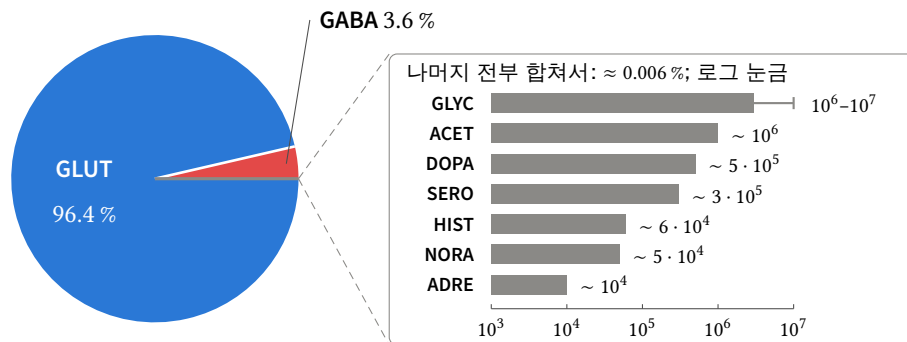
그림 1.2: 표 1.1의 추정치로 본 뇌 속 뉴런 유형의 비율. 원은 거의 전부 GLUT가 차지한다. GABA는 좁은 부채꼴이고, 나머지 유형은 모두 합쳐도 경계선 위의 머리카락 한 올이다. 오른쪽은 그 머리카락을 확대해 뉴런 수를 로그 눈금으로 나타낸 것이다. GLYC의 막대는 범위 10 6 -10 7 의 가운데까지 그렸고, 선분은 범위 전체를 보여 준다. ASPA는 추정치가 없어 그림에 넣지 않았다.
