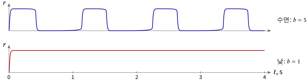
그림 20.2: 두 모드에 있는 같은 무리 (20.2): w = 5 , I = 2 , \theta = 2.5 , \tau = 10 ms, \tau_a = 0.3 s. 피로가 강하면( b = 5 , 서파 수면처럼) 무리는 주기 1.1 s로 활동과 침묵 사이를 오간다(모델의 값; 피질에서 주기는 1초보다 길고, 마취 상태에서는 약 3 s). 피로를 약하게 하면( b = 1 , 아세틸콜린이 이렇게 작용한다) 같은 무리가 고르게 일한다.
