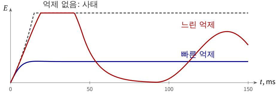
그림 3.4: 입력을 켜 뒤, 되먹임 w_{EE} = 1.5 , \tau_E = 10 ms인 GLUT 무리의 발화율. 억제가 없으면(파선) 활동이 한없이 커진다. 세기 w_{EI}w_{IE} = 2 , \tau_I = 2 ms인 억제가 있으면(파란 곡선) 수준 E^* = h/(1 - 1.5 + 2) = 0.67h 에 자리 잡는다. 억제가 같되 느리면, \tau_I = 30 ms(빨간 곡선), 활동이 진동한다.
