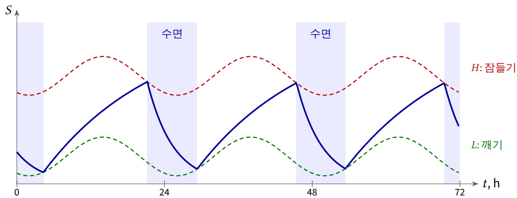
그림 20.1: \tau_r = 18.2 \text{ h} , \tau_d = 4.2 \text{ h} 에서의 수면 압력 S (20.1). 낮에는 S 가 위 문턱값 H 까지 충전되고, 밤에는 (색칠한 부분) 아래 문턱값 L 까지 방전된다. 두 문턱값은 일주기 리듬과 함께 오르내린다. 기계는 스스로 약 16시간 각성, 8시간 수면의 체제에 이른다.
