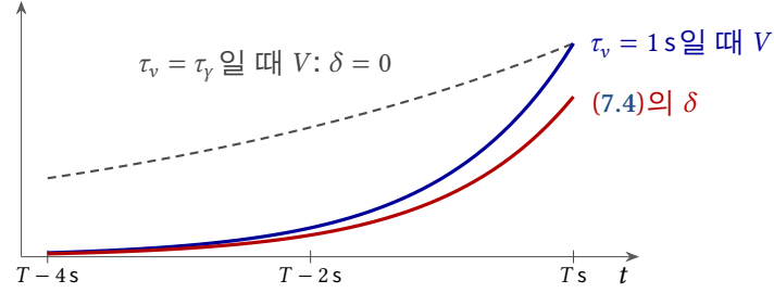
그림 7.2: 보상에 다가갈 때의 도파민 상승을 예측 오차로 본 그림, \tau_\gamma = 4\text{s} . 점선은 지평이 요구하는 그대로 자라는 기대( \delta = 0 ), 파란 선은 더 가파르게 자라는 기대, 빨간 선은 오차 (7.4)이다.
