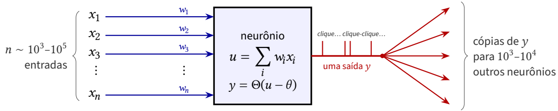
Figura 1.1: O neurônio visto por um engenheiro. Muitas entradas x_i , cada uma com seu peso w_i ; dentro, a soma ponderada u e a comparação com o limiar \theta ( \Theta é o degrau: 1 se o argumento é positivo e 0 caso contrário); uma única saída y , uma sequência de disparos multiplicada por ramificação para milhares de destinatários.
