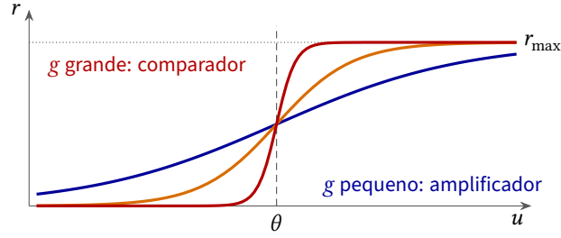
Figura 8.1: Característica de transferência (8.1) com três valores do ganho g .
