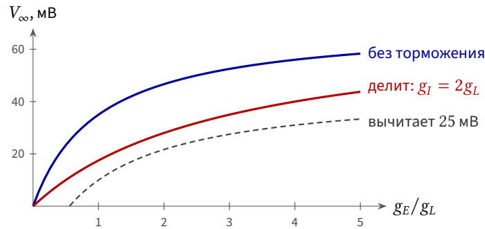
Рис. 3.2: Шунтирующее торможение делит напряжение, а не вычитает из него. Синяя кривая — установившееся напряжение (3.3) без торможения, красная — с тормозящей проводимостью g_I = 2g_L . Красная — та же синяя, растянутая по горизонтали втрое: вход как будто поделили на 1 + g_I/g_L = 3 . Штриховая — торможение, вычитающее постоянные 25 мВ: кривая опускается целиком, наклон не меняется.
