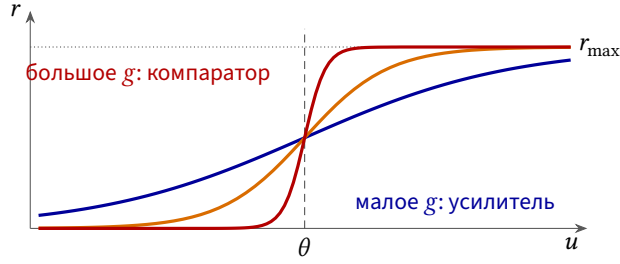
Рис. 8.1: Передаточная характеристика (8.1) при трёх значениях коэффициента усиления g .
