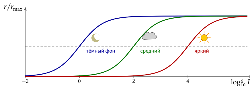
Рис. 11.2: Регулировка усиления датчика света по (11.2). Каждая кривая охватывает два-три порядка яркости; при переходе на более яркий фон \sigma растёт, и кривая сдвигается по логарифмической оси. Вместе сдвигающиеся кривые покрывают весь диапазон.
