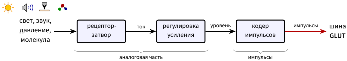
Рис. 11.1: Любой орган чувств как цепь преобразований. Белок-рецептор открывает канал и даёт ток; регулировка усиления приспособляет его к обстановке; кодер (2.1) превращает уровень в импульсы, которые уходят на шину GLUT. В глазу и ухе первые каскады вообще не выдают импульсов: сигнал остаётся аналоговым, пока не приходится передавать его далеко.
