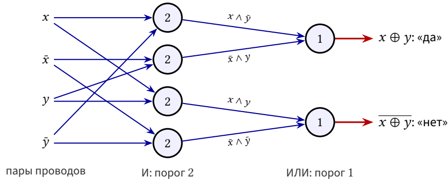
Рис. 2.2: Исключающее ИЛИ на двухпроводном коде, только из GLUT-нейронов. Число в кружке — порог в единицах веса одного входа. Четыре нейрона И узнают четыре сочетания входов, два нейрона ИЛИ собирают их в пару проводов ответа.
