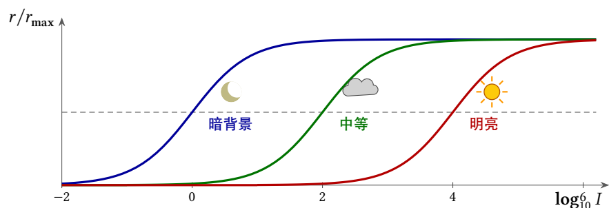
图 11.2: 按式 (11.2) 进行的光传感器增益调节。每条曲线覆盖两三个数量级的亮度；换到更亮的背景时 \sigma 增大，曲线沿对数轴移动。这些移动的曲线合起来覆盖整个范围。
