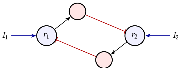
图 3.3: 二选一。两群 GLUT 神经元（蓝）经 GABA 中介（红）相互抑制。
