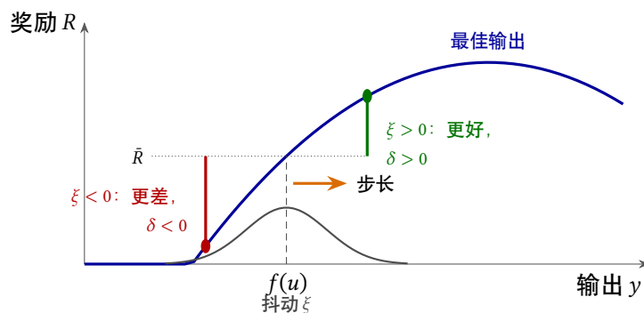
图 6.3: 噪声即搜索 (6.6)。神经元的输出在 f(u) 附近抖动。向右的随机偏离 (绿色) 得到的比预期多, \delta > 0 ; 向左的 (红色) 得到的少, \delta < 0 。两种情况下乘积 \delta\xi 都是正的, 权重向右移动, 即向奖励增大的方向。平均而言, 步长与斜率 R' 成正比: 在山顶, 向两侧的偏离同样糟糕, 步长相互抵消。
