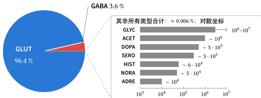
图 1.2: 按表 1.1 的估计, 各类神经元在脑中所占的比例。圆几乎全被 GLUT 占满; GABA 是一个窄扇区, 其余所有类型合起来只是边界上的一根细线。右侧把这根细线放大, 按神经元数的对数坐标画出; GLYC 的柱子画到 10^6 - 10^7 区间的中点, 横线段表示整个区间。ASPA 没有估计值, 图中未画出。
