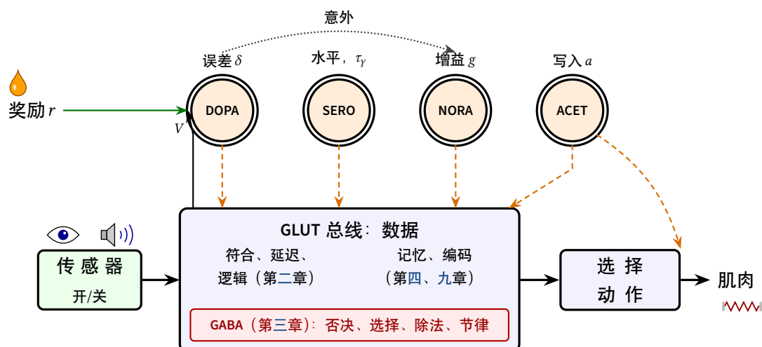
图 10.1: 整台机器。GLUT 总线把数据从传感器送到动作选择；GABA 控制总线内部的数据流。双线圆圈是广播通道；虚线箭头表示把它们的信号发给整个网络，每条通道有自己的旋钮。DOPA 接收奖励 r 和来自总线内部评论器的预期 V （第 6 章）；点线箭头是一个假说：NORA 通过异常大的误差得知意外（第 8 章）。
