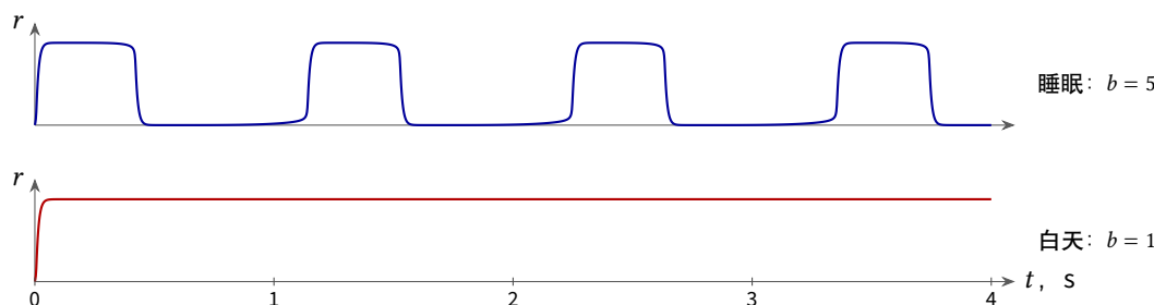
图 20.2: 同一个群体 (20.2) 在两种模式下: w = 5 , I = 2 , \theta = 2.5 , \tau = 10 ms, \tau_a = 0.3 s。疲劳强时 ( b = 5 , 如同慢波睡眠), 群体在工作和静默之间摆动, 周期为 1.1 s (模型值; 皮层中周期超过一秒, 麻醉下约为 3 s)。减弱疲劳 ( b = 1 ) ——乙酰胆碱就是这样起作用的——同一个群体便平稳地工作。
