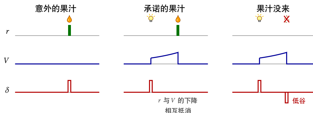
图 6.4: 误差 (6.8) 的三种情况；自上而下依次为奖励 r 、期望 V 和误差 \delta 。左：没有期望，果汁完全出乎意料。中：灯使 V 跃升，这是 dV/dt 的跃变， \delta 的爆发落在灯亮时。之后 V 恰好按视野的要求增长， \delta = 0 ；果汁到来时，奖励 r 与 V 的下降相互抵消。右： V 在没有奖励时下降——低谷。这就是图 1.4 中的爆发、转移和低谷，只是现在能看出它们从何而来。
