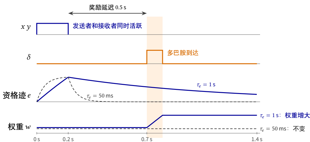
图 6.2: 按规则 (6.5) 的资格迹。共同活动持续 0.2 \text{ s} , 多巴胺在其结束半秒后到达。资格迹以各自最大值的比例表示。慢的资格迹 ( \tau_e = 1 \text{ s} ) 此刻仍然存在, 快的 ( \tau_e = 50 \text{ ms} ) 早已消退。
