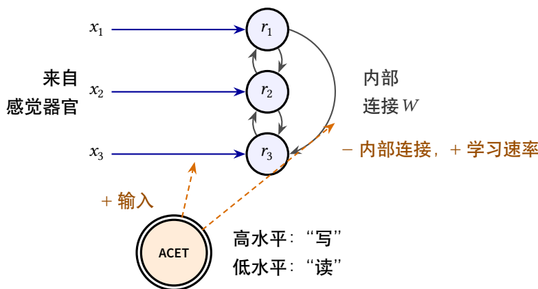
图 9.1: ACET 作为写使能线。神经元 r_i 从感觉器官接收输入 x_i (蓝色箭头), 并通过存有模式的内部连接 W (灰色) 相互兴奋。乙酰胆碱 (虚线箭头) 增强输入、削弱内部连接并使权重更容易改变, 如 (9.1) 所示。
