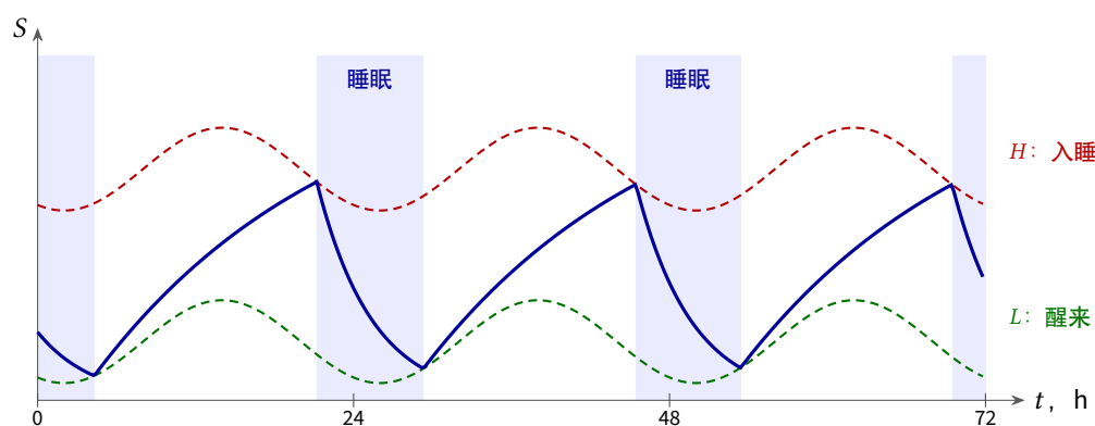
图 20.1: \tau_r = 18.2 \text{ h} 、 \tau_d = 4.2 \text{ h} 时的睡眠压力 S (20.1)。白天 S 充电到上阈值 H ，夜里（阴影部分）放电到下阈值 L ；两个阈值都随昼夜节律摆动。机器自己进入大约 16 小时清醒、8 小时睡眠的模式。
