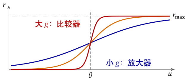
图 8.1: 增益 g 取三个值时的传递特性 (8.1)。
