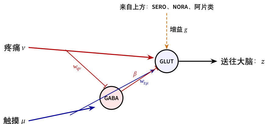
图 14.1: 按模型 (14.2) 的脊髓疼痛闸门。输出 GLUT 神经元接收疼痛 v 和来自触摸 \mu 的微弱兴奋。抑制性中间神经元 (GABA 或 GLYC) 被触摸兴奋, 并按闸门理论的假设被疼痛关闭。增益 g 经广播通道从上方到来。
