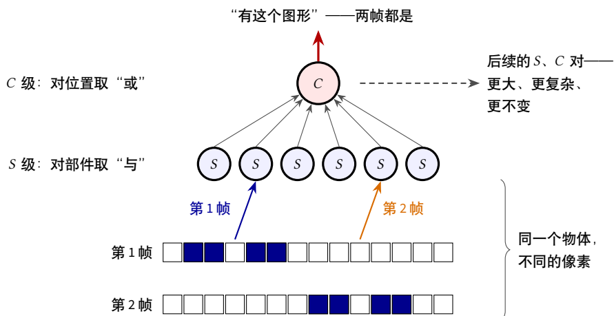
图 12.1: 流水线中的一对级。S 神经元在不同位置寻找同一个部件组合；只要在任何地方找到它，C 神经元就作出响应 (12.1)。第 1 帧和第 2 帧中的图形激活不同的 S 神经元，却激活同一个 C 神经元。后续的级对在越来越大、越来越复杂的组合上重复同样的操作。
