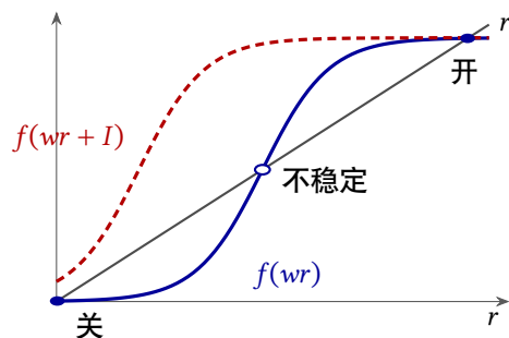
图 2.5: 由强反馈 GLUT 神经元群构成的存储单元。实线是没有外部驱动的情形：与直线 r 有两个稳定交点（“关”和“开”），中间还有一个不稳定交点。短暂的驱动 I （虚线）只留下上面那个交点。
