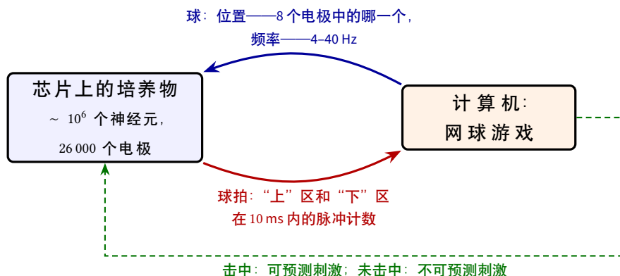
图 22.1: DishBrain 回路。蓝色箭头是输入：球的位置用位置编码和频率编码表示（第 4 章）。红色箭头是输出：两个区的计数之差移动球拍。绿色虚线是每个回合之后的反馈，也是试验台上唯一的“老师”。
