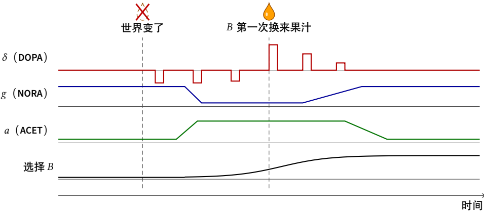
图 10.2: 一个事件穿过整台机器的全过程。这是依据第 六-九 章的模型和假说画出的定性示意图，而不是计算结果。变化之后 DOPA 以低谷作答；按照假说，反复的低谷抬高意外信号，NORA 降低增益，ACET 开启写入；B 第一次换来果汁时出现爆发，选择转向 B，各旋钮随后复原。
