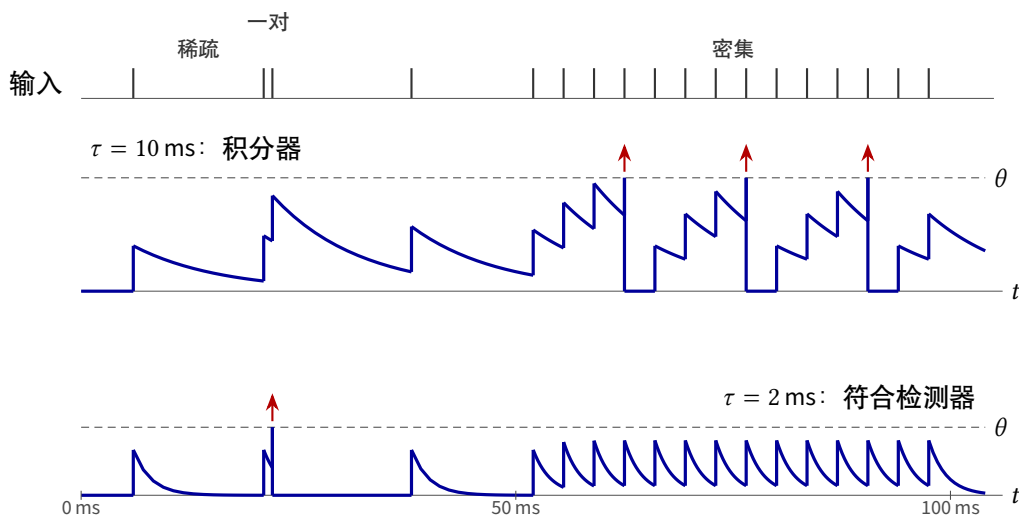
图 4.3: 同一个输入，两种不同的接收者。每个脉冲把电压抬高 w ，之后电压像神经元模型 (2.1) 那样回落；红色箭头是接收者的脉冲。慢接收者 ( \tau = 10 \text{ ms} , \theta = 2.5w ) 在脉冲多的地方发放，注意不到那一对。快接收者 ( \tau = 2 \text{ ms} , \theta = 1.5w ) 只对窗口 (2.2) 内的一对脉冲发放，而放过密集却不符合的脉冲流。
