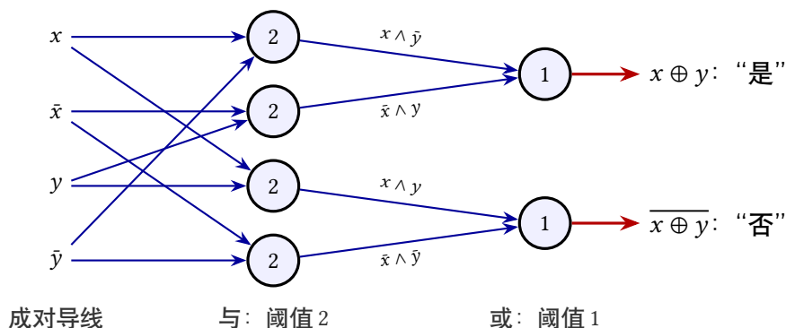
图 2.2: 用双线编码、仅由 GLUT 神经元实现的异或。圆圈中的数是以单个输入权重为单位的阈值。四个与神经元识别输入的四组组合，两个或神经元把它们汇集成一对答案导线。
