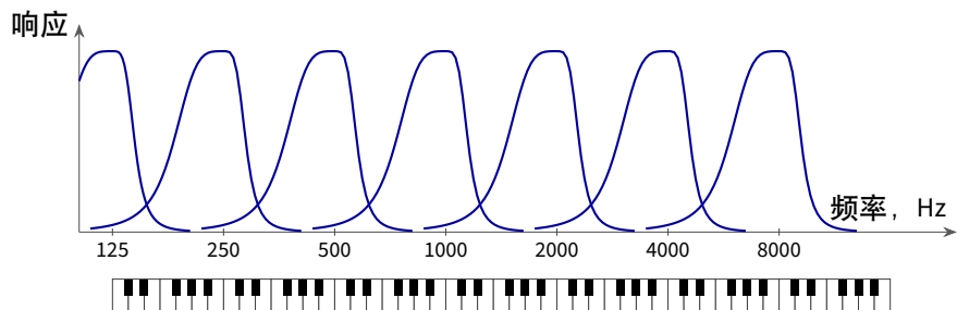
图 11.3: 耳朵作为带通滤波器组的示意图。每条曲线是某一段上的传感器对不同频率声音的响应；中心频率相隔一个倍频程，就像对数刻度上的琴键。真实滤波器的高频侧陡峭，低频侧平缓。下方是键盘：与耳朵一样，每个倍频程在上面占据相同的位置。
