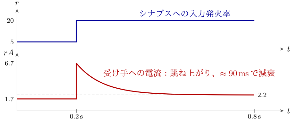
図 4.4: 式 (4.6) による枯渇するシナプス、 U = 0.5 、 \tau_{\text{rec}} = 0.8 \text{ s} 。電流は毎秒 A_0 単位で表し、破線は定常電流である。定常電流は 1.7 から 2.2 に増えただけだが、跳躍の瞬間には 6.7 に達する。シナプスが受け手に伝えるのは、発火率がいくらかではなく、発火率が変わったということである。
