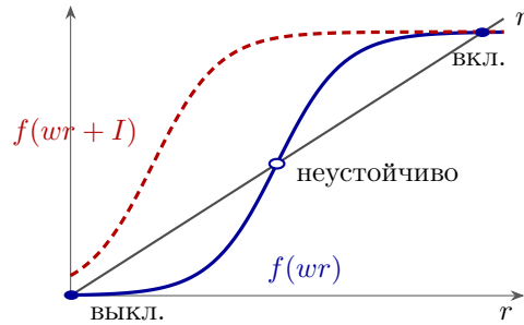
Рис. 2.5: Память из группы GLUT -нейронов с сильной обратной связью. Сплошная кривая — без внешнего притока: два устойчивых пересечения с прямой r , «выключено» и «включено», и неустойчивое между ними. Короткий приток I (штриховая кривая) оставляет только верхнее.
