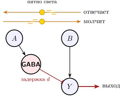
Рис. 3.1: Детектор направления движения. B возбуждает Y , A тормозит его через GABA -посредника с задержкой d . При движении от A к B со скоростью около \Delta x/d торможение гасит возбуждение; при обратном движении оно опаздывает. Жёлтое пятно с чёрточками — свет, бегущий над датчиками.
